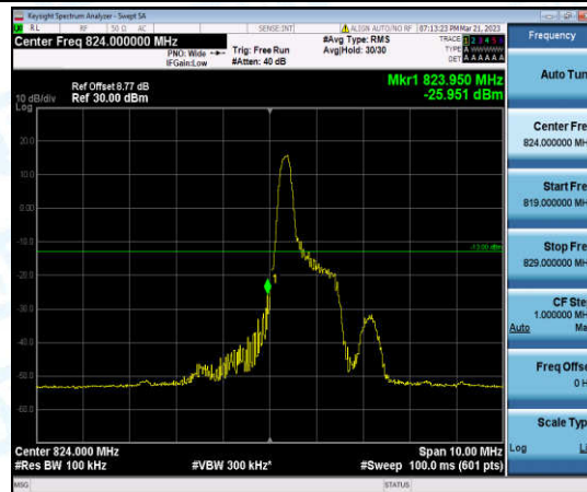
Band5-5MHz-16QAM-20425-1-0-Low--25.95-PASS
