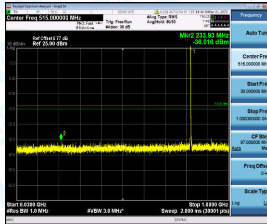
Band5-5MHz-QPSK-20425-1-0-Low-30-1000--36.02-PASS
