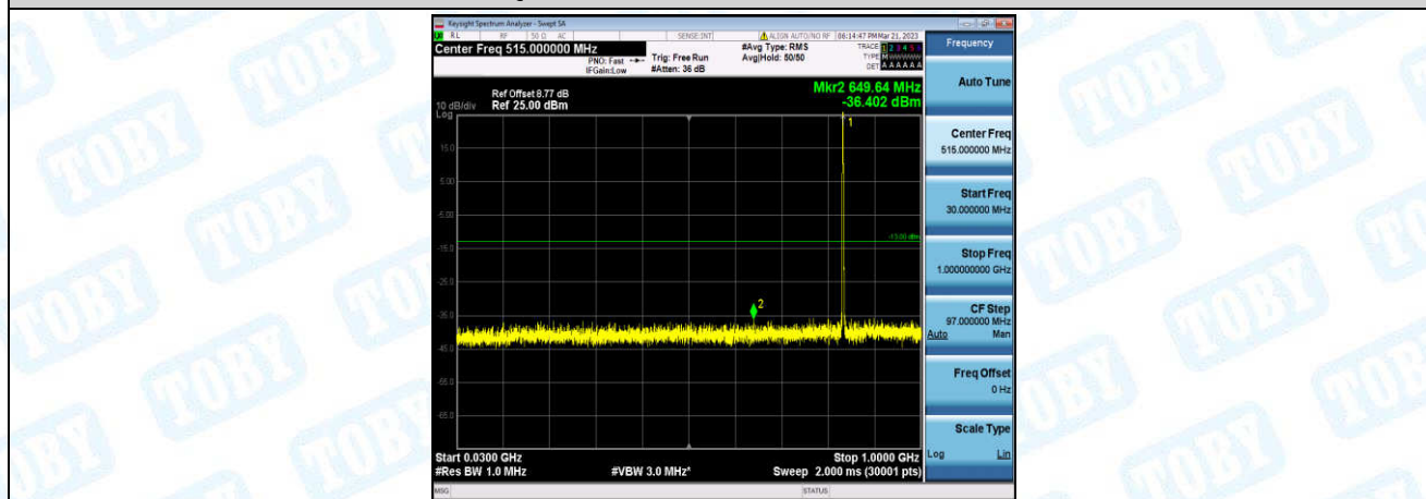
Band5-1.4MHz-QPSK-20525-1-0-Low-30-1000--36.4-PASS
