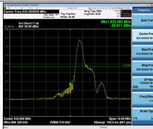
Band5-10MHz-QPSK-20450-1-0-Low--35.61-PASS
