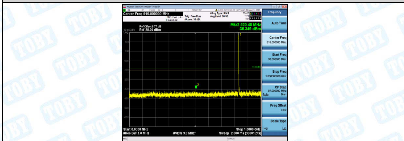
Band5-5MHz-QPSK-20525-1-0-Low-30-1000--35.35-PASS
