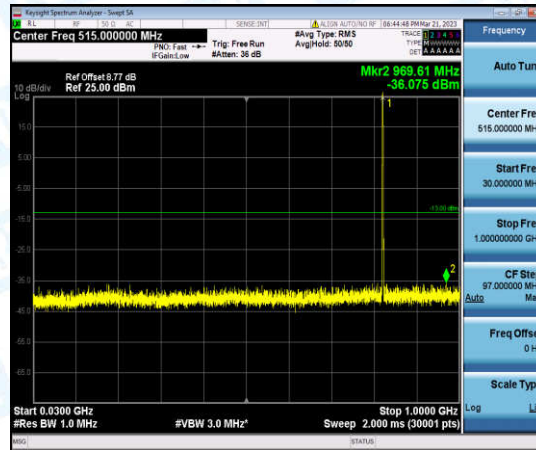
Band5-3MHz-16QAM-20415-1-0-Low-30-1000--36.08-PASS
