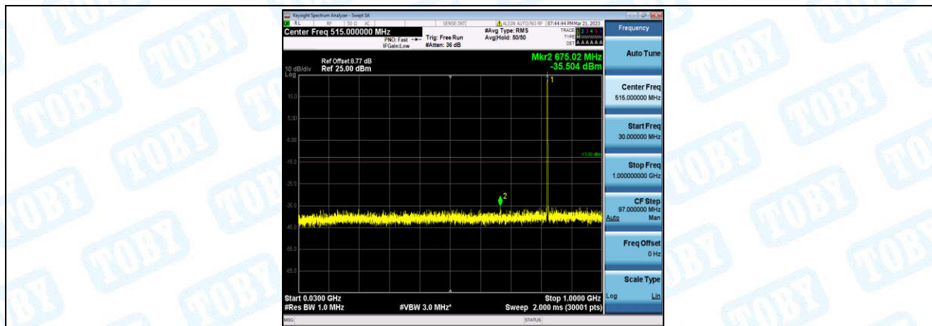
Band5-10MHz-QPSK-20450-1-0-Low-30-1000--35.5-PASS
