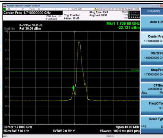
Band66-20MHz-QPSK-132072-1-0-Low--33.13-PASS
