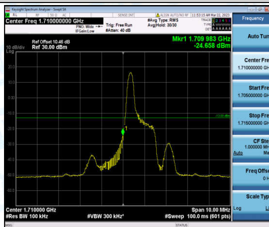
Band66-5MHz-QPSK-131997-1-0-Low--24.66-PASS
