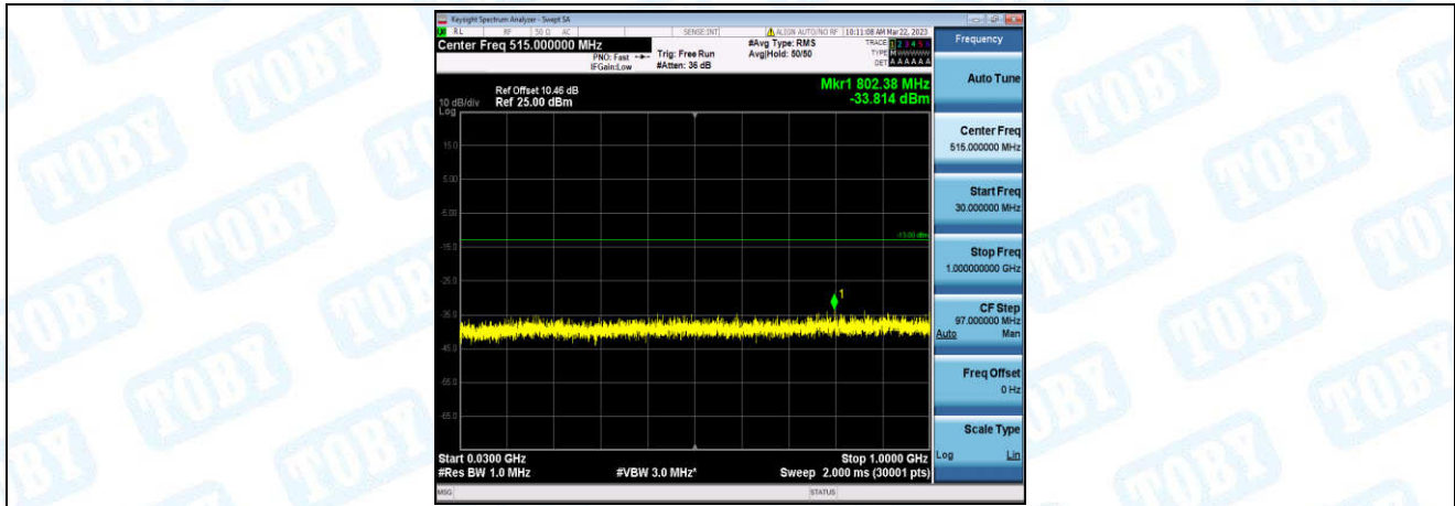
Band66-3MHz-QPSK-131987-1-0-Low-30-1000--33.81-PASS
