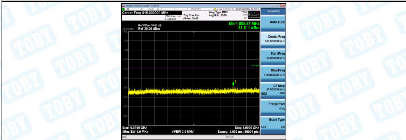
Band66-5MHz-QPSK-132322-1-0-Low-30-1000--33.51-PASS
