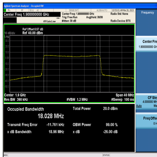
Band2-20MHz-16QAM-19100-100RB#0-18.028
