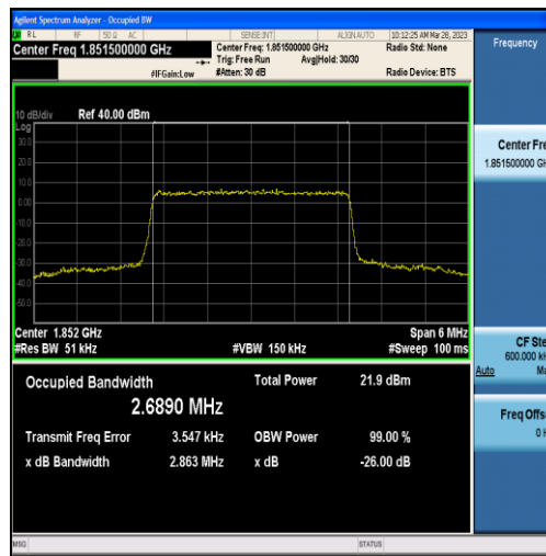
Band2-3MHz-QPSK-18615-15RB#0-2.6890
