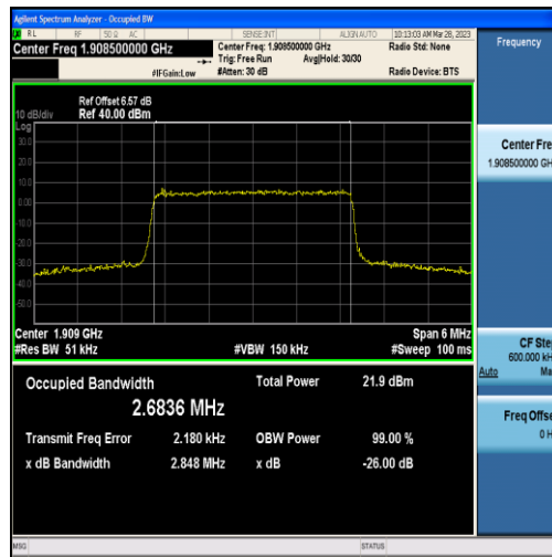
Band2-3MHz-QPSK-19185-15RB#0-2.6836
