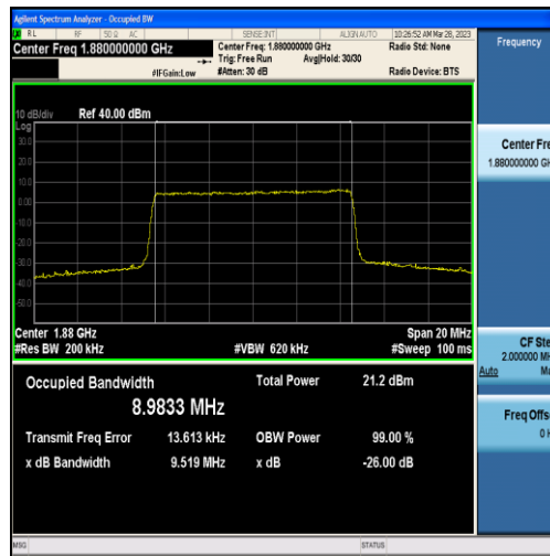
Band2-10MHz-QPSK-18900-50RB#0-8.9833
