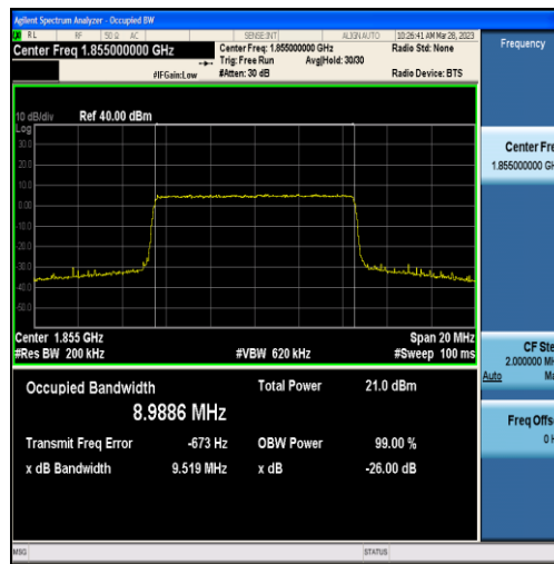
Band2-10MHz-QPSK-18650-50RB#0-8.9886
