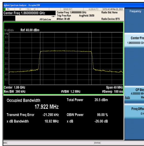
Band2-20MHz-QPSK-18700-100RB#0-17.922
