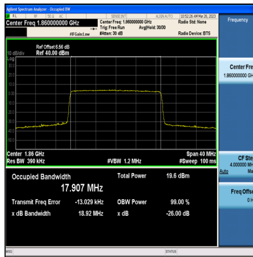
Band2-20MHz-16QAM-18700-100RB#0-17.907
