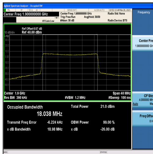
Band2-20MHz-QPSK-19100-100RB#0-18.038
