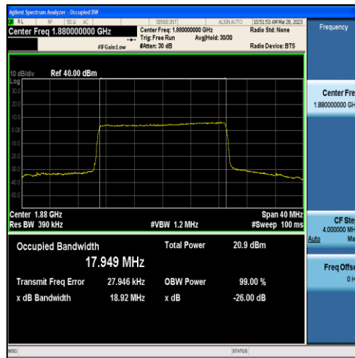
Band2-20MHz-QPSK-18900-100RB#0-17.949
