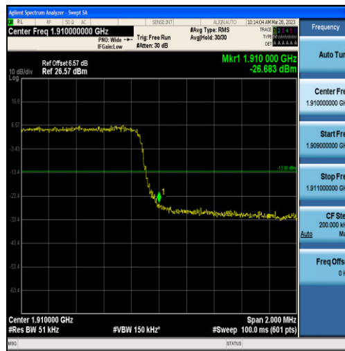
Band2-3MHz-QPSK-19185-15RB#0
