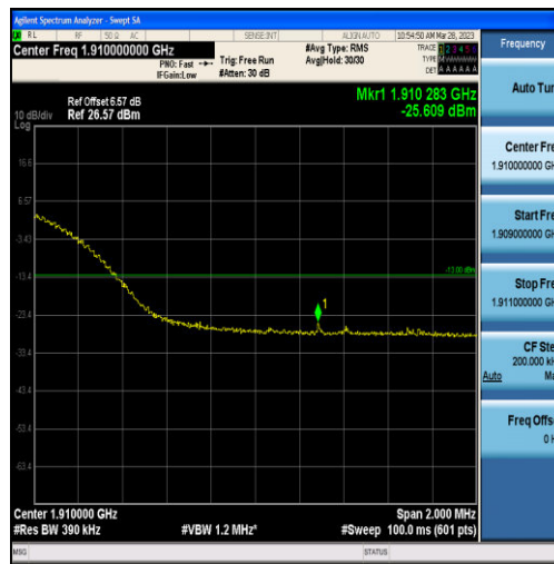
Band2-20MHz-QPSK-19100-100RB#0
