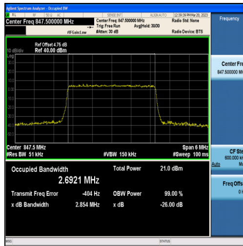
Band5-3MHz-QPSK-20635-15RB#0-2.6921
