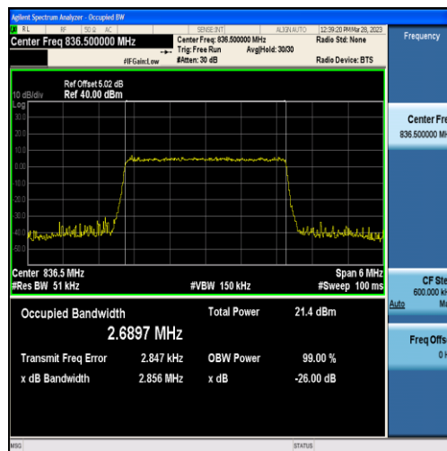
Band5-3MHz-QPSK-20525-15RB#0-2.6897
