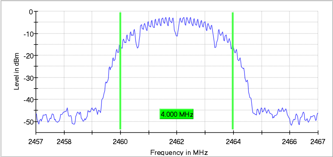
Mode 1 / CH10 (2462 MHz)
