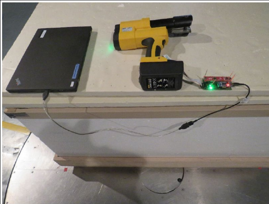
EUT Test Setup (horizontal)
