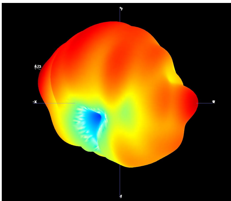
B1.2 2442MHz
