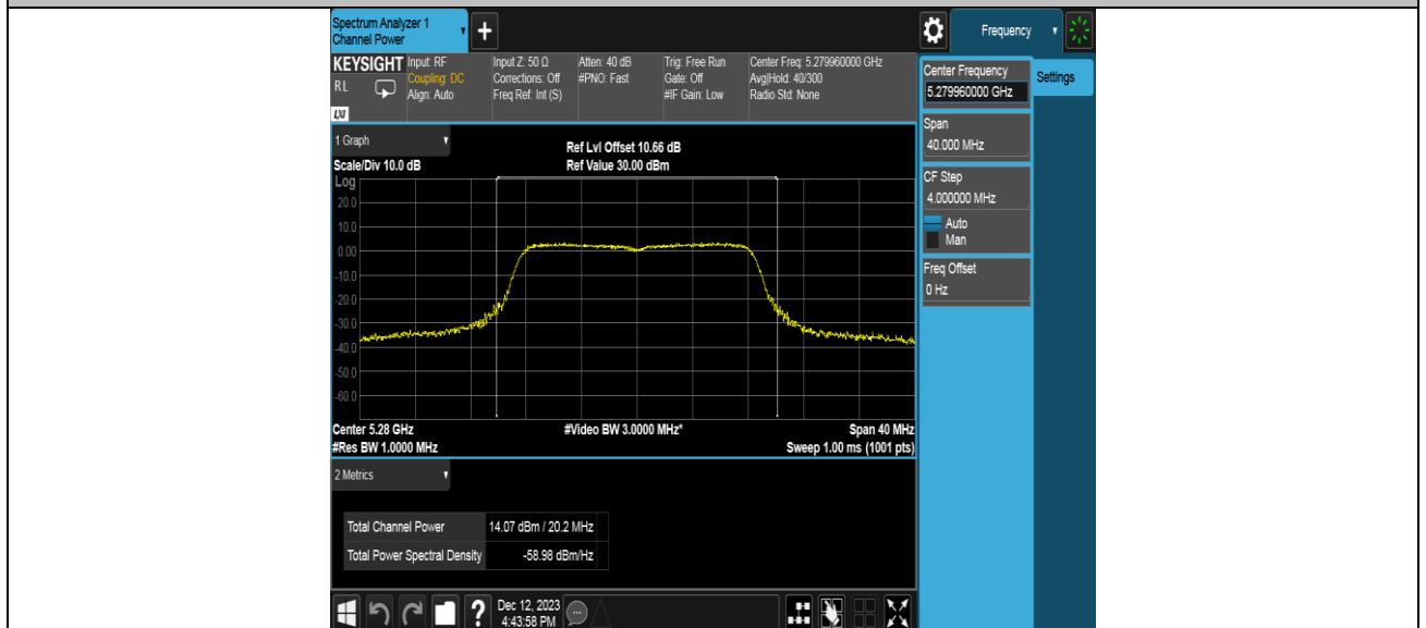
11A_Ant1_5280
