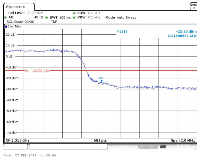
Band40-10MHz-QPSK-38750-1RB#0
