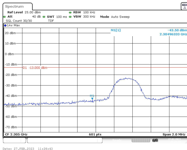
Band40-5MHz-QPSK-38725-25RB#0
