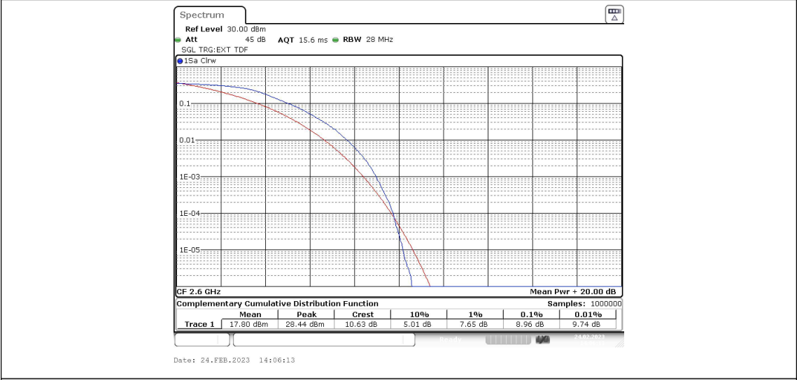
Band41-20MHz-QPSK-41140-1RB#0
