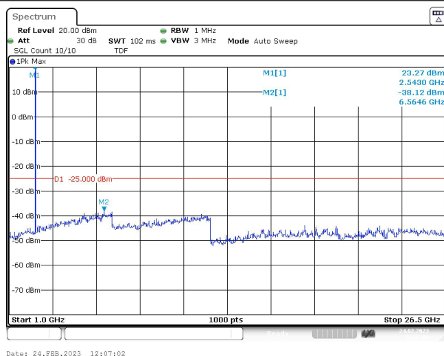
Band41-5MHz-QPSK-40265-1RB#0-Range2:1000~26500MHz
