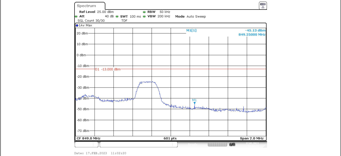
Band5-3MHz-QPSK-20635-1RB#14
