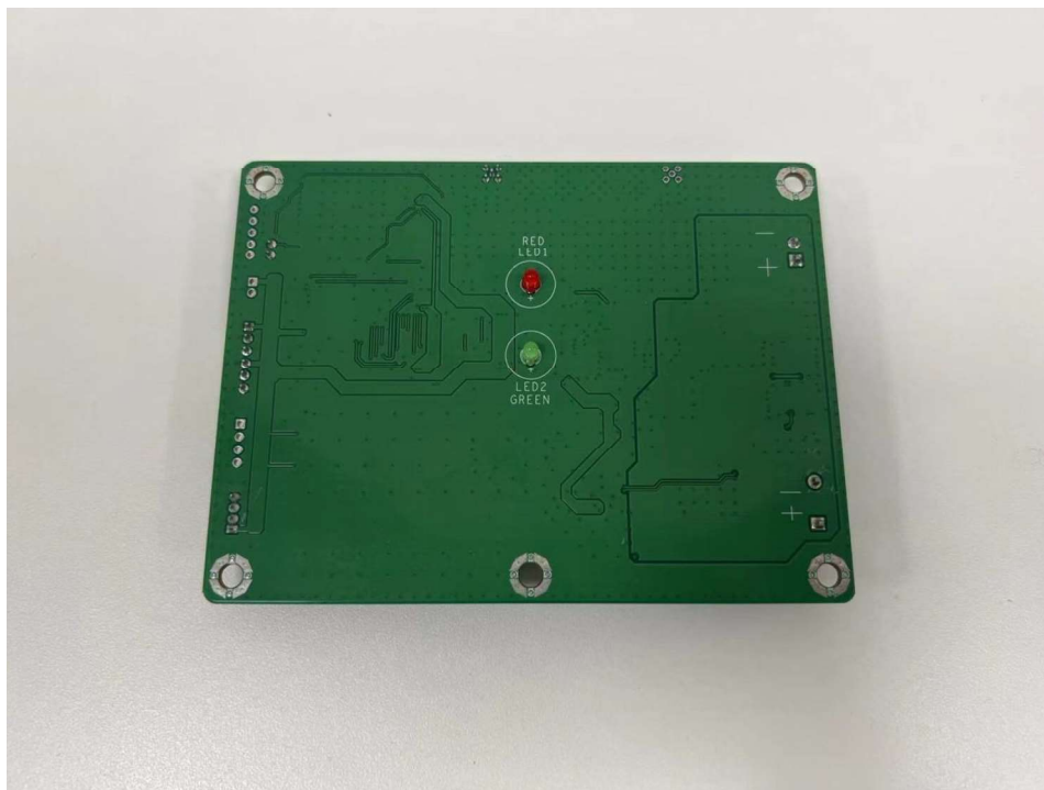
Internal: Bottom
