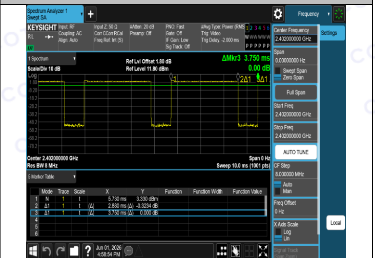
NTNV-2DH5-Ant1-2402
