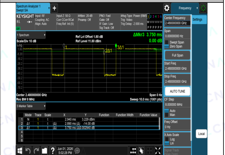
NTNV-2DH5-Ant1-2480
