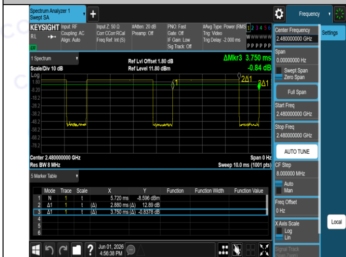
NTNV-DH5-Ant1-2480
