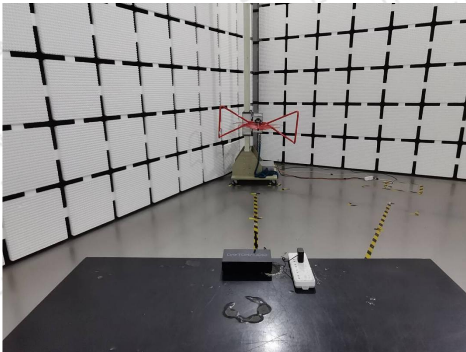
30MHz-1000MHz
