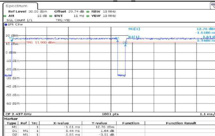
11AX40MIMO Ant0 2437
