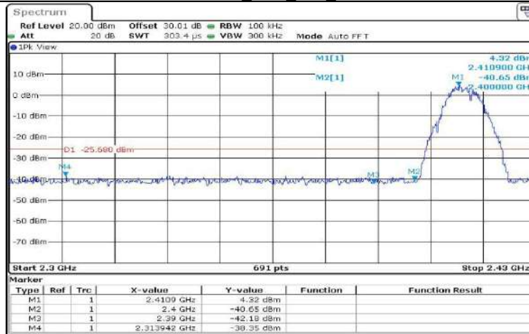
11B-CDD_Ant0_Low_2412
