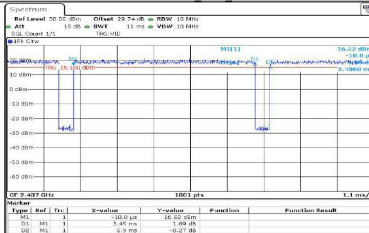
11AX20MIMO_Ant0_2437
