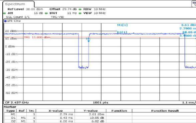
11N40MIMO Ant0 2437
