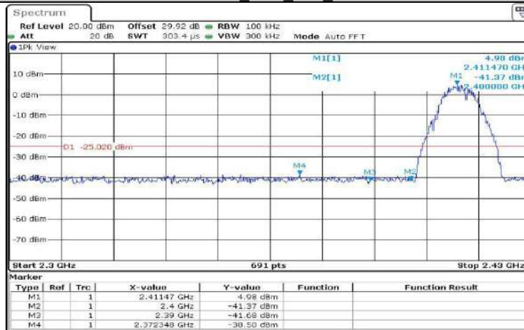
11B-CDD_Ant1_Low_2412
