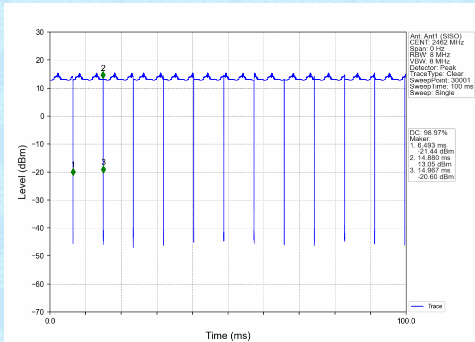
802.11b_HCH_2462MHz_Ant1 (SISO)_NTNV
