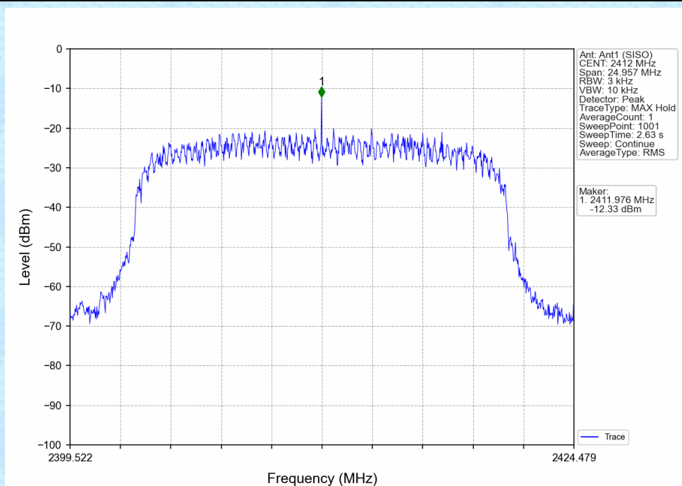
802.11n(HT20)_LCH_2412MHz_Ant1 (SISO)_NTNV
