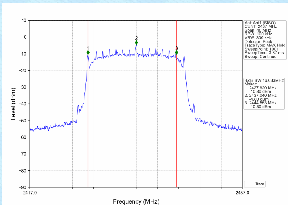
802.11n(HT20)_MCH_2437MHz_Ant1 (SISO)_NTNV
