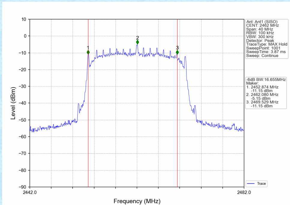
802.11n(HT20)_HCH_2462MHz_Ant1 (SISO)_NTNV
