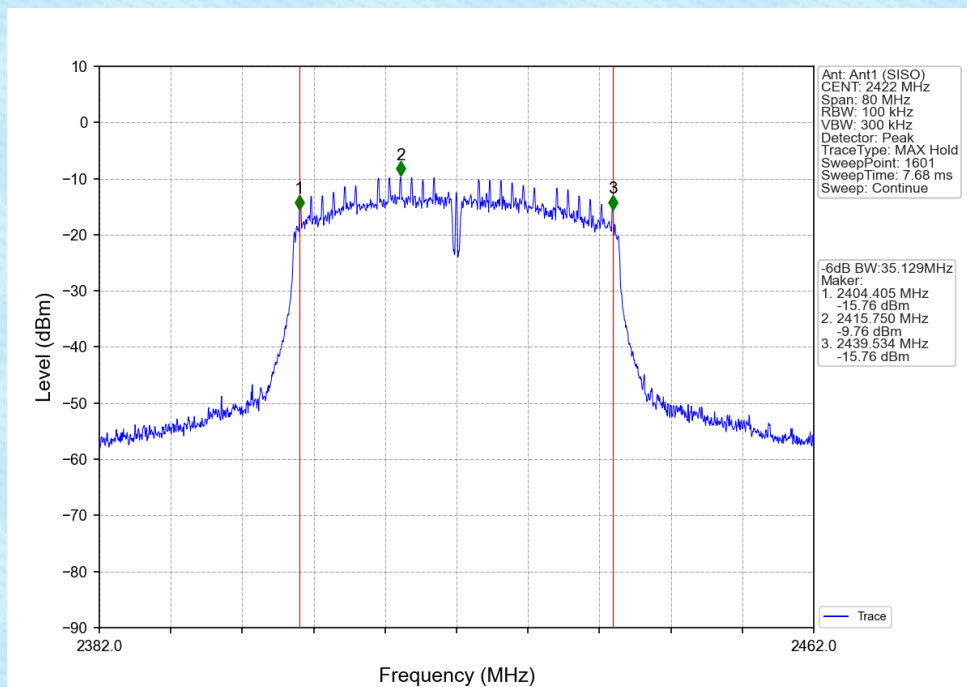
802.11n(HT40)_LCH_2422MHz_Ant1 (SISO)_NTNV
