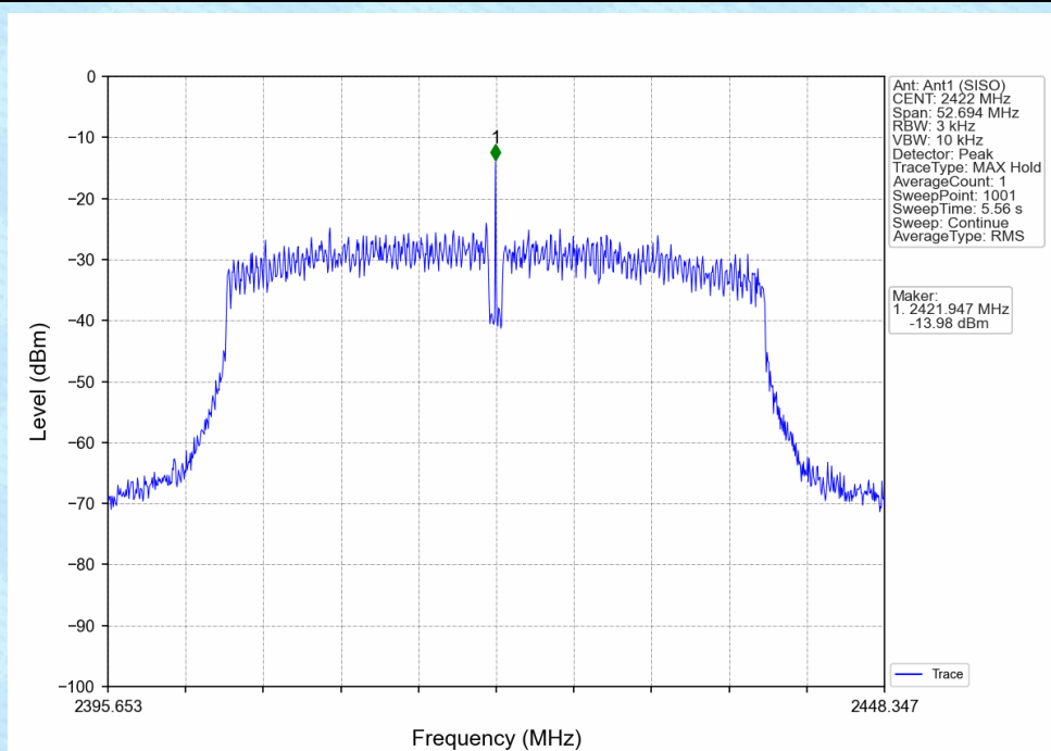
802.11n(HT40)_LCH_2422MHz_Ant1 (SISO)_NTNV
