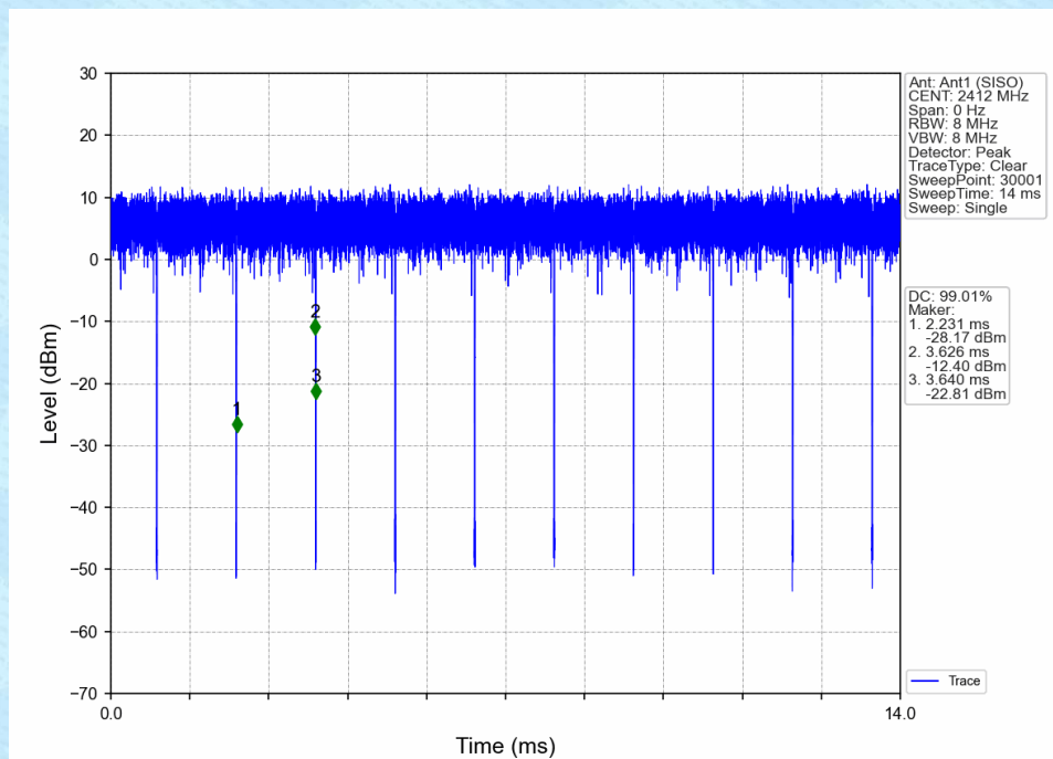
802.11g_LCH_2412MHz_Ant1 (SISO)_NTNV
