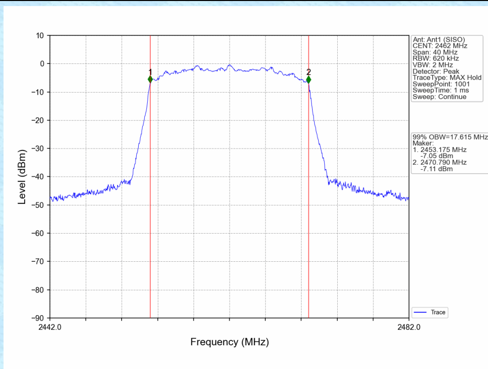
802.11g_HCH_2462MHz_Ant1 (SISO)_NTNV
