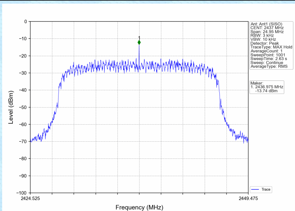
802.11n(HT20)_MCH_2437MHz_Ant1 (SISO)_NTNV
