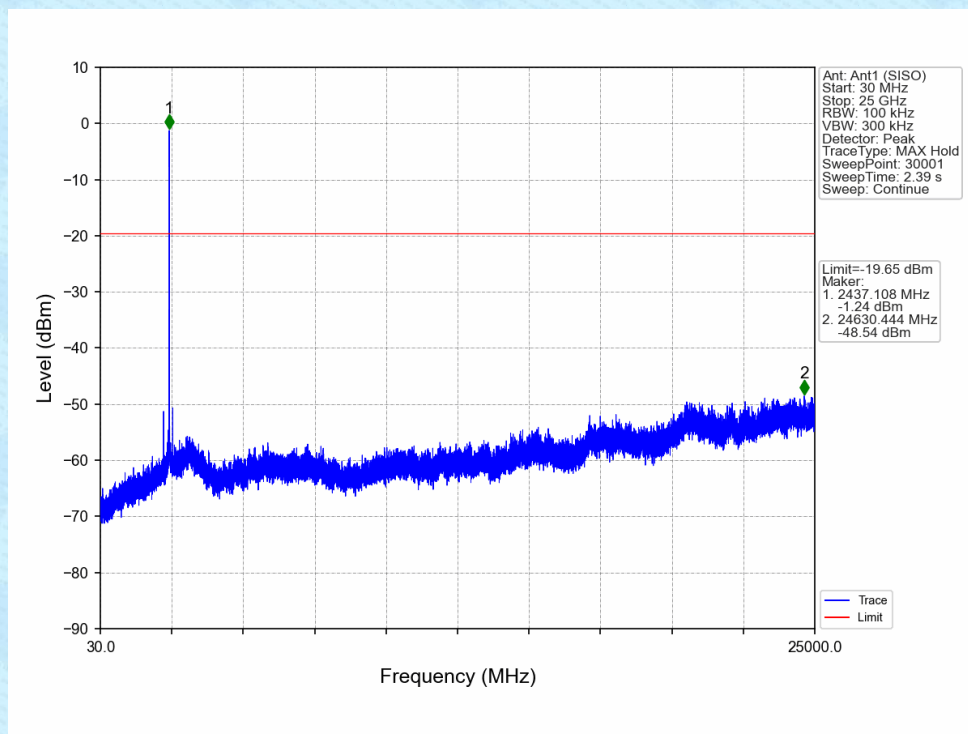
802.11b_MCH_2437MHz_Ant1 (SISO)_NTNV
