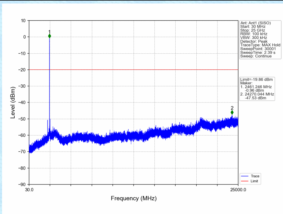
802.11b_HCH_2462MHz_Ant1 (SISO)_NTNV
