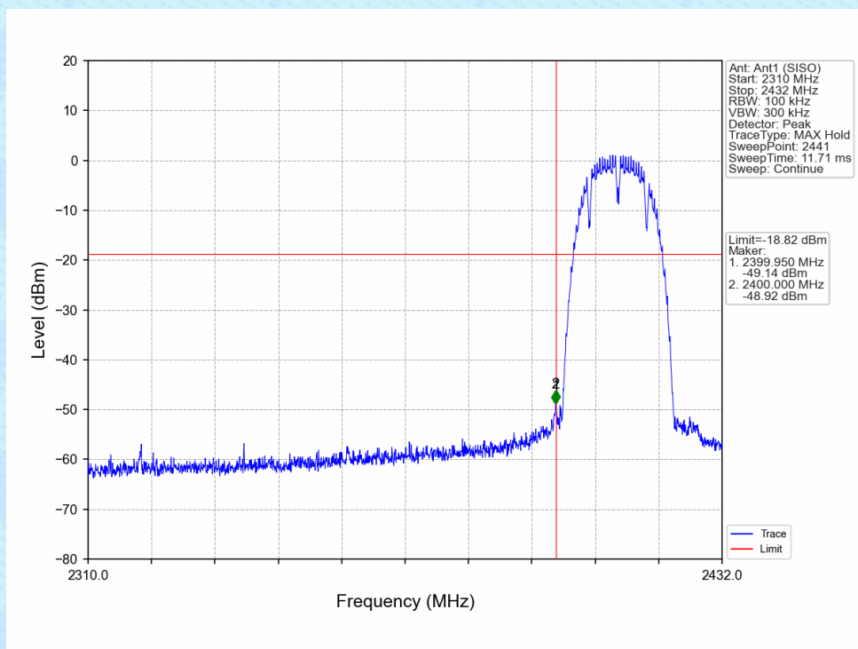
802.11b_LCH_2412MHz_Ant1 (SISO)_NTNV
