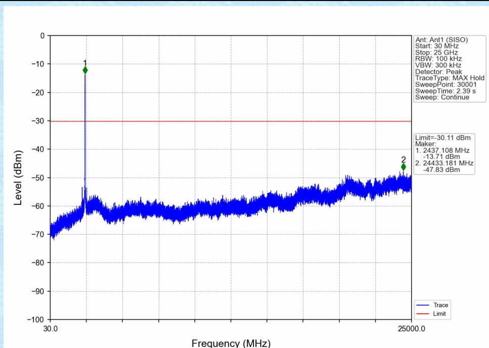
802.11n(HT40)_MCH_2437MHz_Ant1 (SISO)_NTNV
