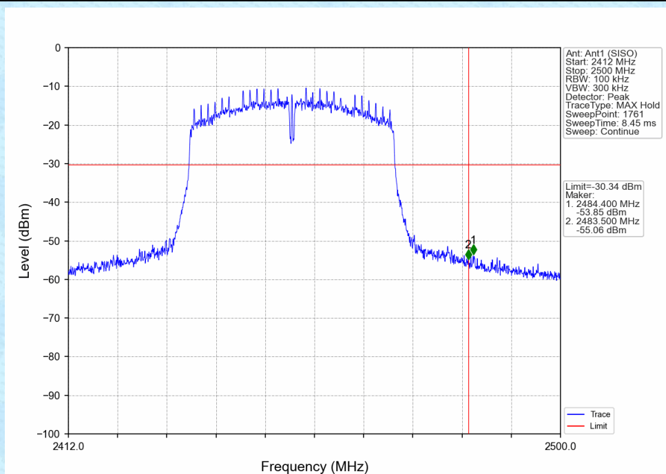
802.11n(HT40)_HCH_2452MHz_Ant1 (SISO)_NTNV
