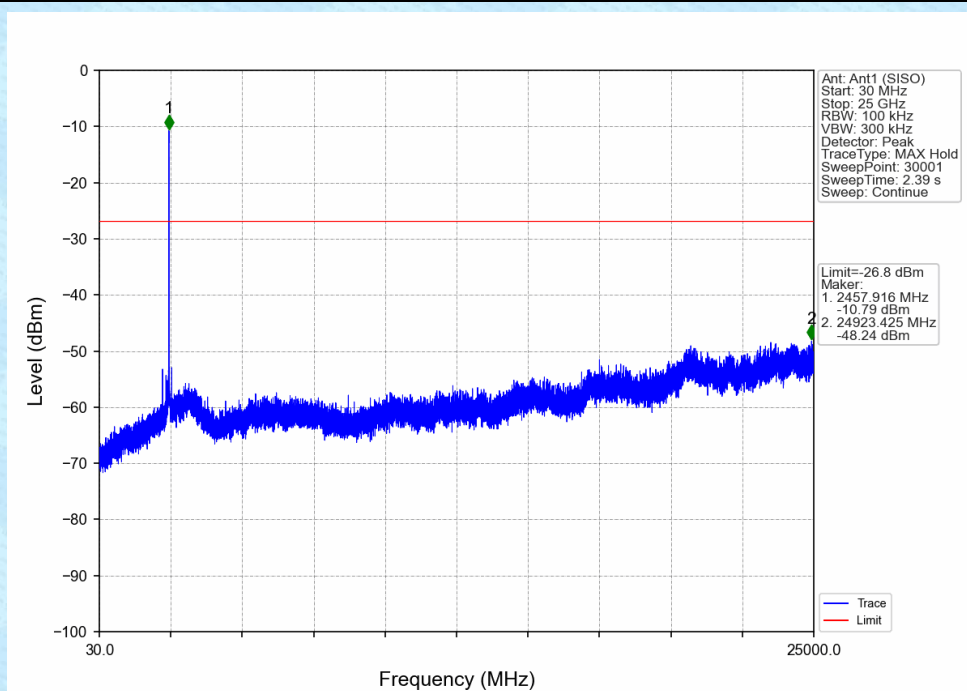
802.11g_HCH_2462MHz_Ant1 (SISO)_NTNV
