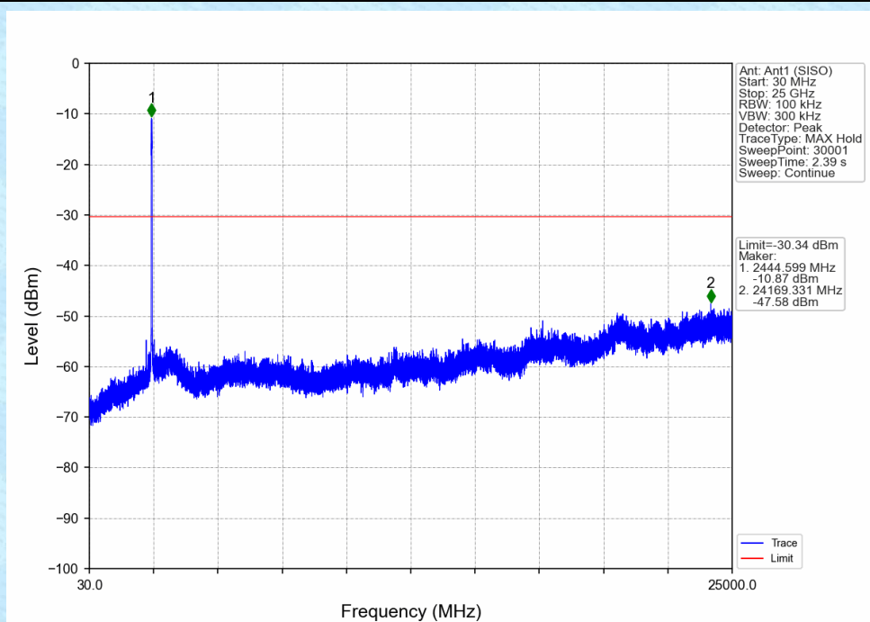
802.11n(HT40)_HCH_2452MHz_Ant1 (SISO)_NTNV
