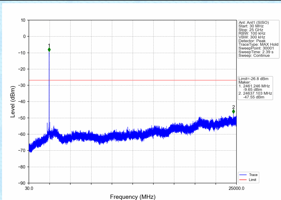
802.11g_HCH_2462MHz_Ant1 (SISO)_NTNV
