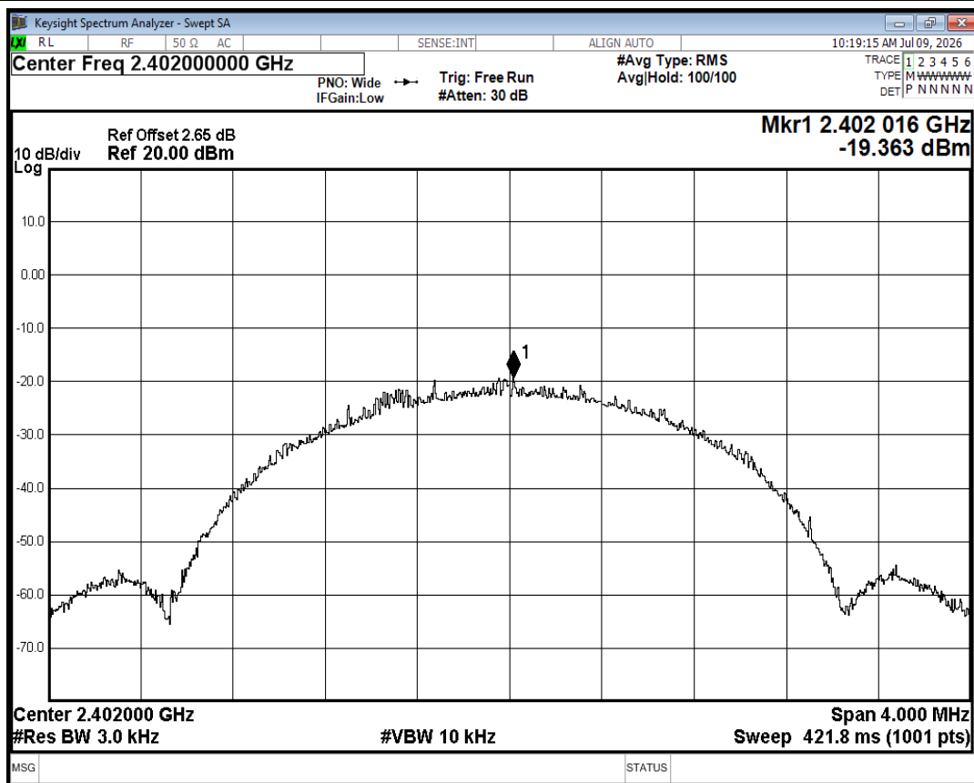
PSD NVNT BLE 2M 2402MHz Ant1
