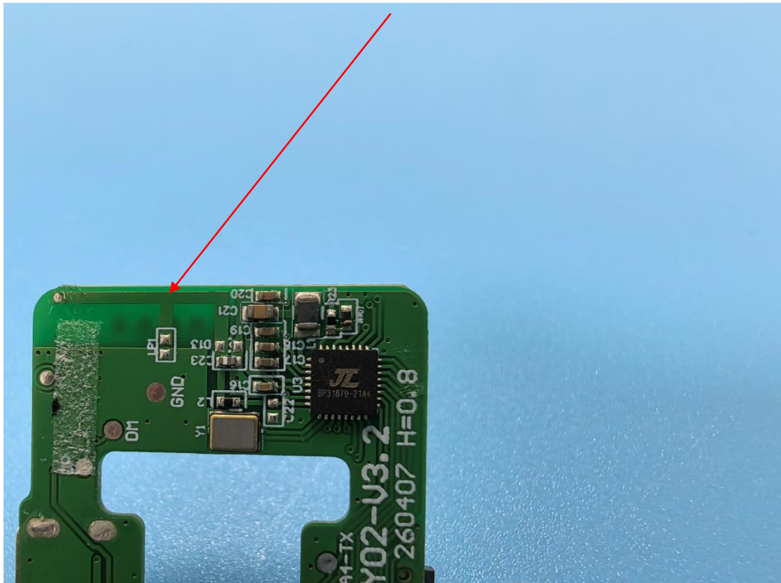
BLE Antenna
