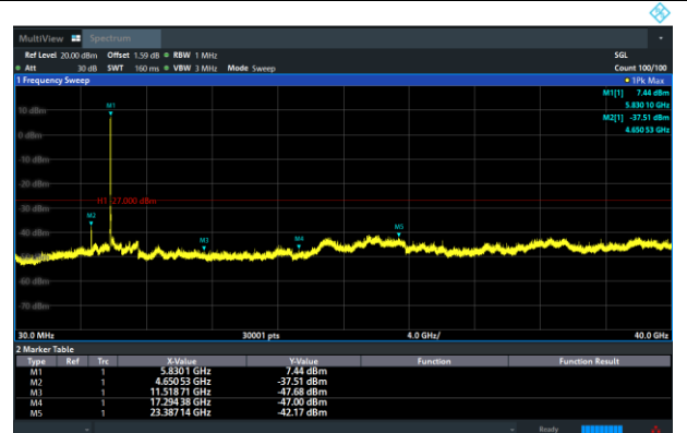
11ax(HE40) CH159
