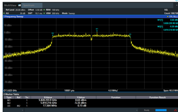
11ac(HT20) CH165
