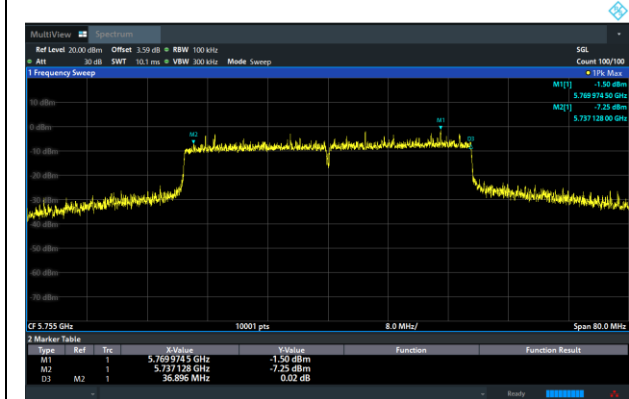
11ax(HE40) CH151
