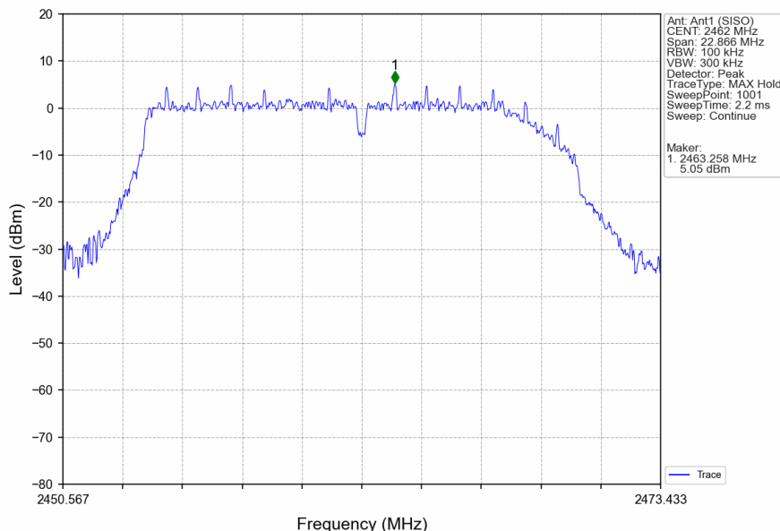
802.11g_HCH_2462MHz_Ant1 (SISO)_NTNV
