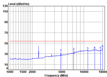
11b_TX_CH_06_Vertical-Avg
