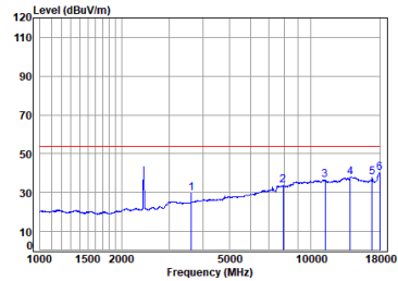
11n_20M_TX_CH_01_Vertical-Avg
