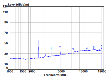
11b_TX_CH_06_Horizontal-Avg
