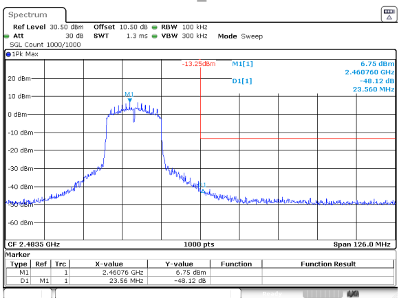
802.11n20_2462MHz
