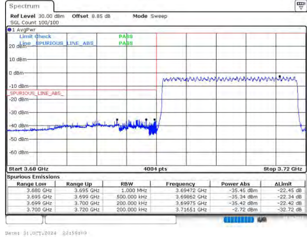
n77(3700-3980) SCS=30kHz DFT_16QAM BW=20MHz LowChannel=647334 RB=50@0
