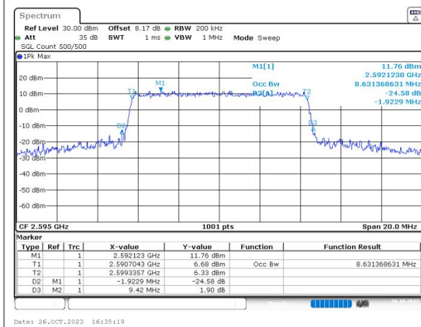
n38 SCS=30kHz CP_QAM16 BW=10MHz Channel=519000 RB=24@0
