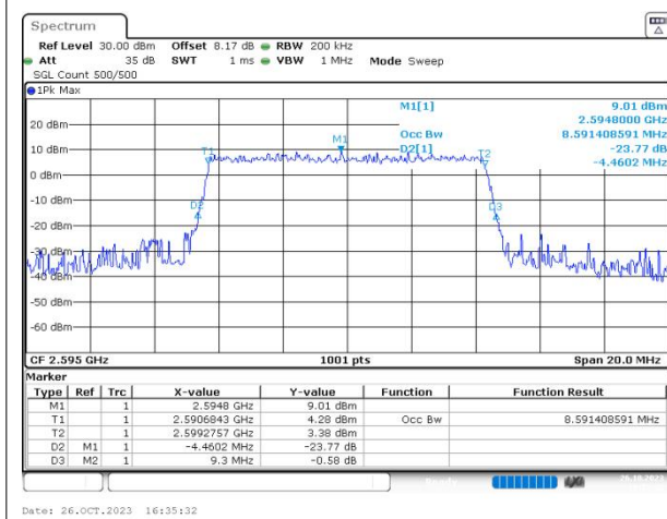
n38 SCS=30kHz CP_QAM256 BW=10MHz Channel=519000 RB=24@0
