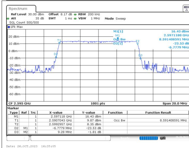
n38 SCS=30kHz DFT_BPSK BW=10MHz Channel=519000 RB=24@0
