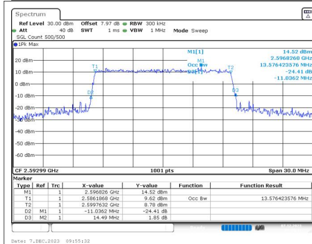
n41 SCS=30kHz CP_QPSK BW=15MHz Channel=518598 RB=38@0
