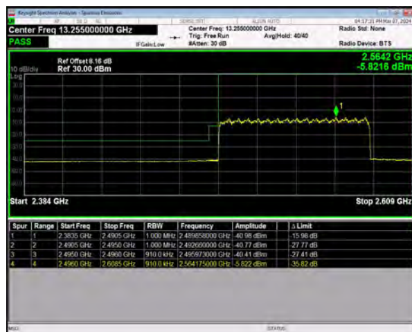
n41 SCS=30kHz DFT_64QAM BW=90MHz
