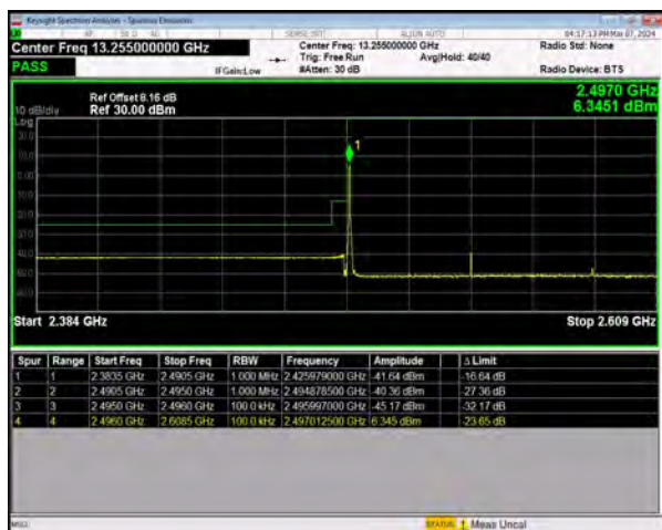
n41 SCS=30kHz DFT_64QAM BW=90MHz
