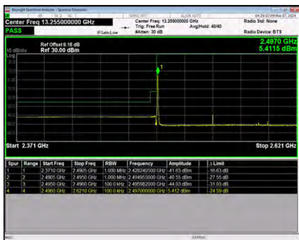
n41 SCS=30kHz DFT_64QAM BW=100MHz
