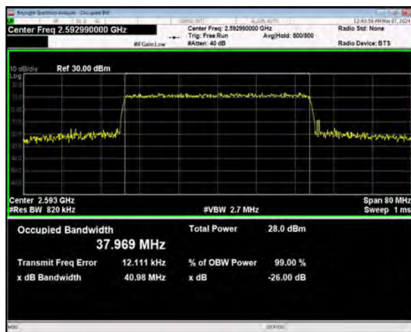
n41 SCS=30kHz CP_QPSK BW=40MHz Channel=518598 RB=106@0
