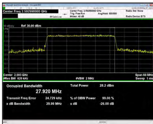
n41 SCS=30kHz CP_16QAM BW=30MHz Channel=518598 RB=78@0
