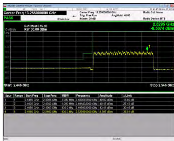
n41 SCS=30kHz DFT_256QAM BW=40MHz
