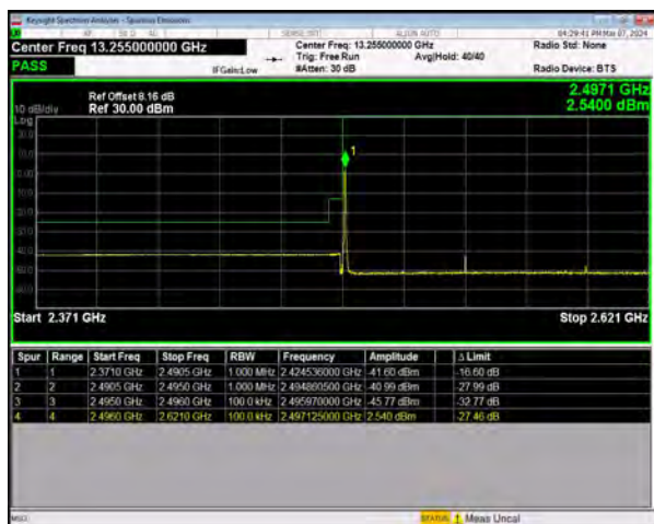
n41 SCS=30kHz DFT_256QAM BW=100MHz
