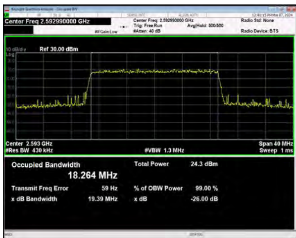
n41 SCS=30kHz CP_256QAM BW=20MHz Channel=518598 RB=51@0
