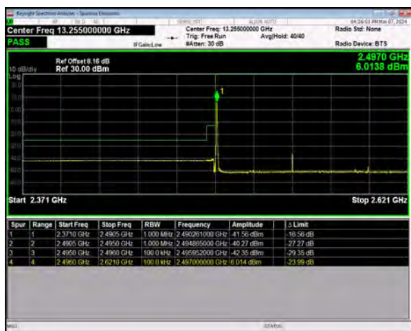
n41 SCS=30kHz DFT_16QAM BW=100MHz
