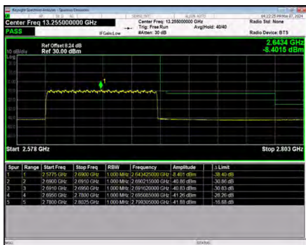
n41 SCS=30kHz DFT_256QAM BW=90MHz
