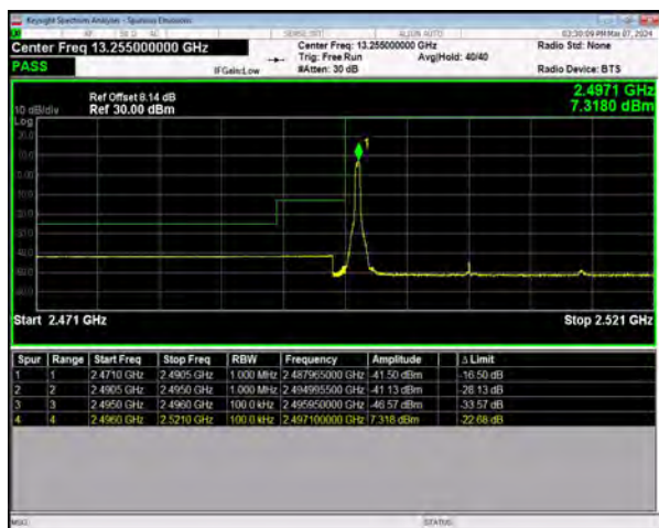
n41 SCS=30kHz DFT_64QAM BW=20MHz
