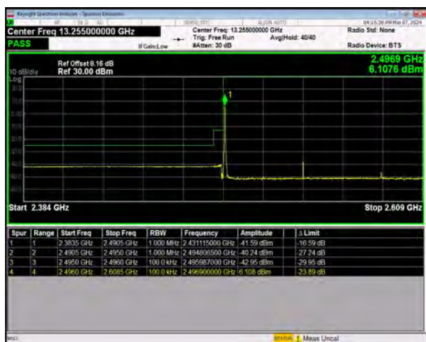
n41 SCS=30kHz DFT_16QAM BW=90MHz
