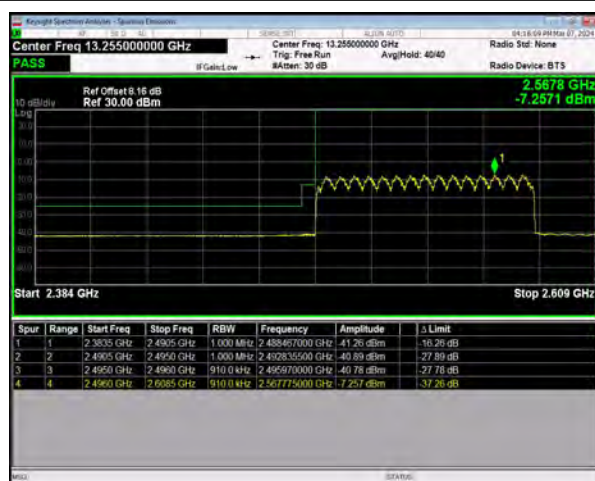
n41 SCS=30kHz DFT_256QAM BW=90MHz
