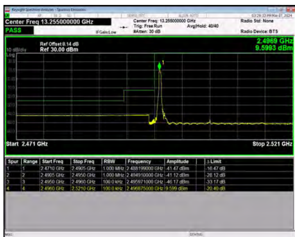
n41 SCS=30kHz DFT_16QAM BW=20MHz
