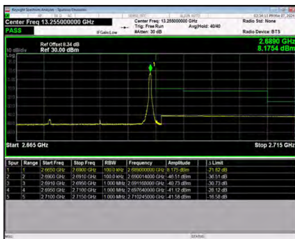
n41 SCS=30kHz DFT_64QAM BW=20MHz
