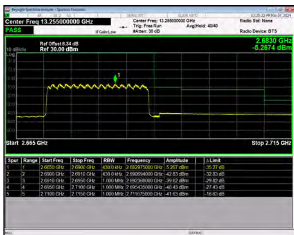
n41 SCS=30kHz DFT_256QAM BW=20MHz
