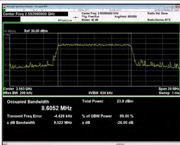
n41 SCS=30kHz CP_256QAM BW=10MHz Channel=518598 RB=24@0
