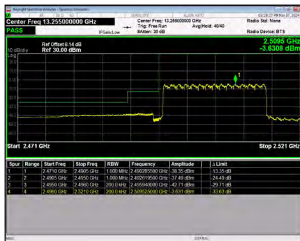
n41 SCS=30kHz DFT_BPSK BW=20MHz LowChannel=501204 RB=50@0
