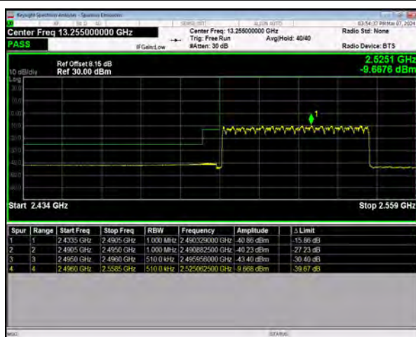
n41 SCS=30kHz DFT_256QAM BW=50MHz
