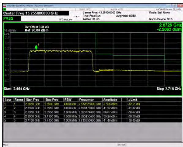
n41 SCS=30kHz DFT_BPSK BW=20MHz HighChannel=535998 RB=50@0
