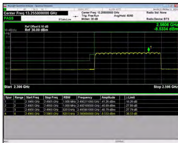
n41 SCS=30kHz DFT_256QAM BW=80MHz
