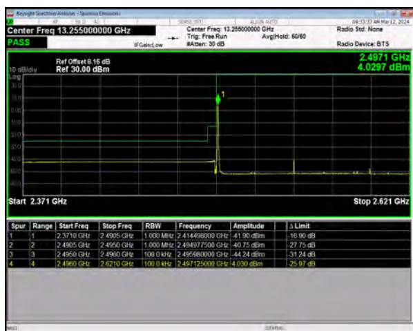
n41 SCS=30kHz DFT_16QAM BW=100MHz
