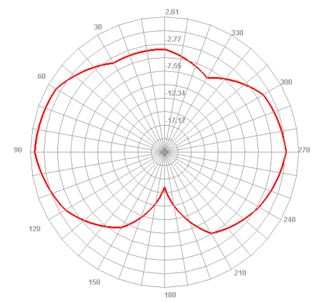
2450.000MHz E2
