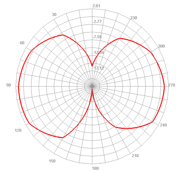
2450.000MHz E1
