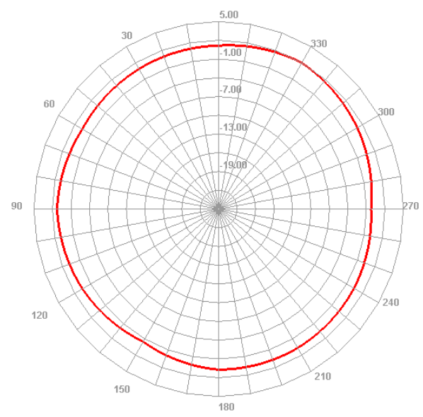
2450.000MHz H
