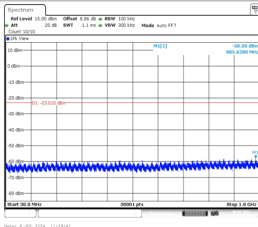
11G-Ant1-2412-30~1000-PASS
