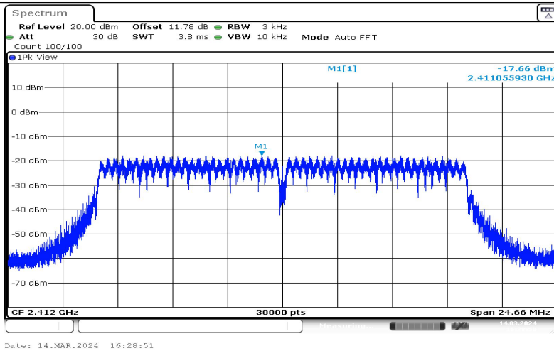
11G-Ant1-2412--17.66-0.00-0.00-0.00
