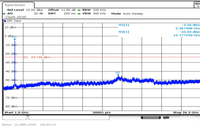
11N20SISO-Ant1-2462-1000~26500--3.74
