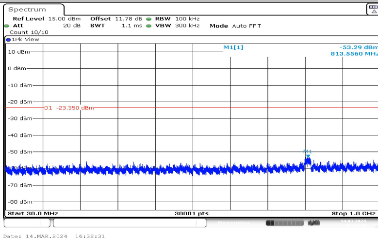
11G-Ant1-2437-30~1000--3.35
