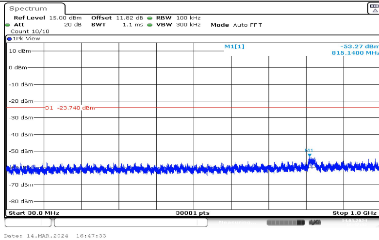
11N20SISO-Ant1-2462-30~1000--3.74
