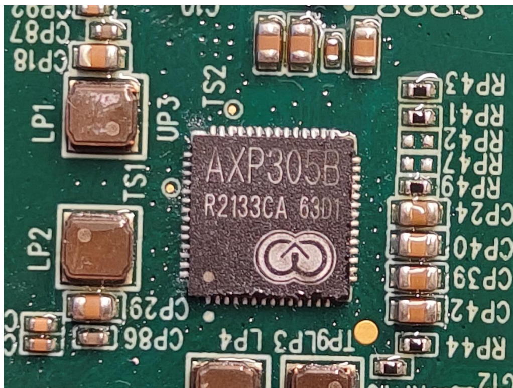
(36) EUT Photo
