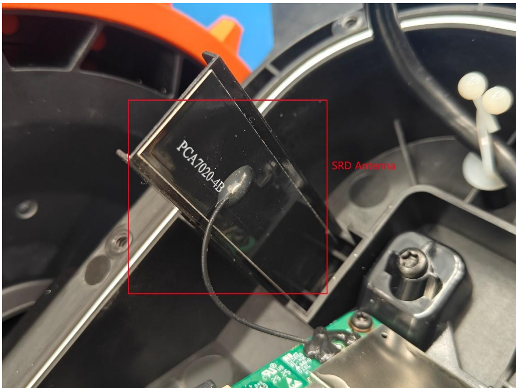
(40) EUT Photo
