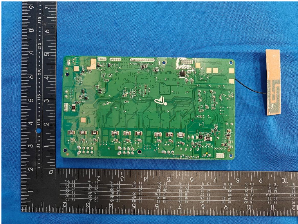
(47) EUT Photo
