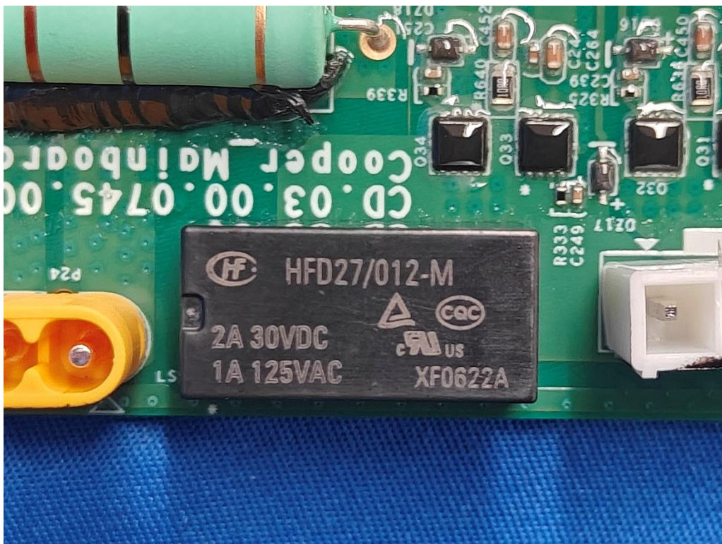
(46) EUT Photo
