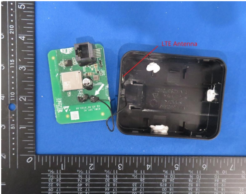
(6) EUT Photo
