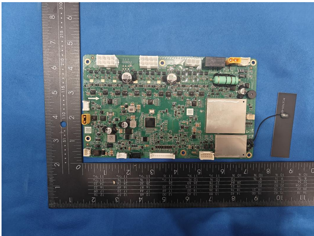
(40) EUT Photo
