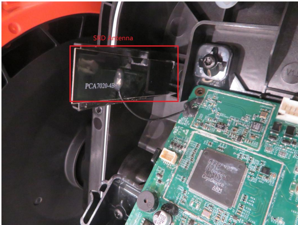
(40) EUT Photo
