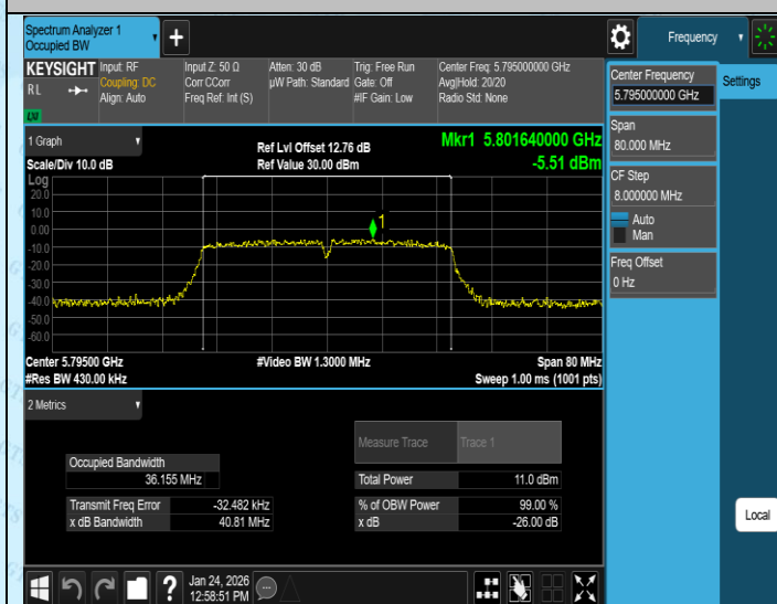
11AC40MIMO-Ant1-5795
