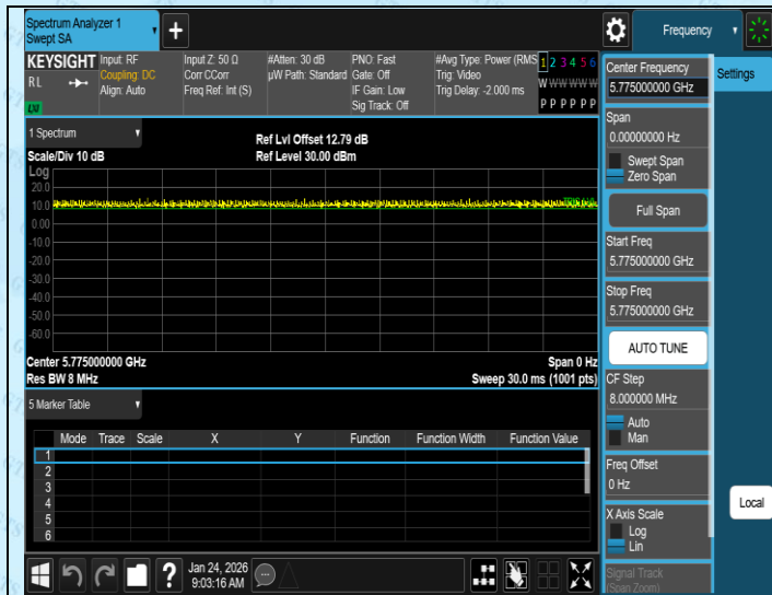
NTNV-11AC80SISO-Ant1-5775
