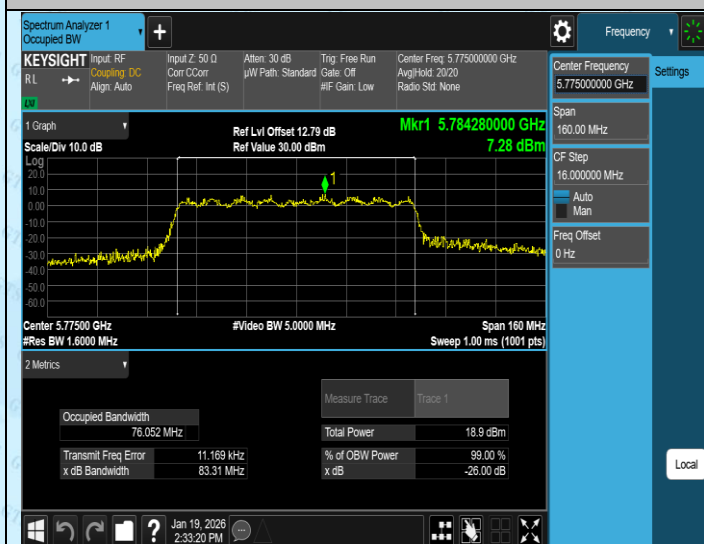
11AC80SISO-Ant3-5775
