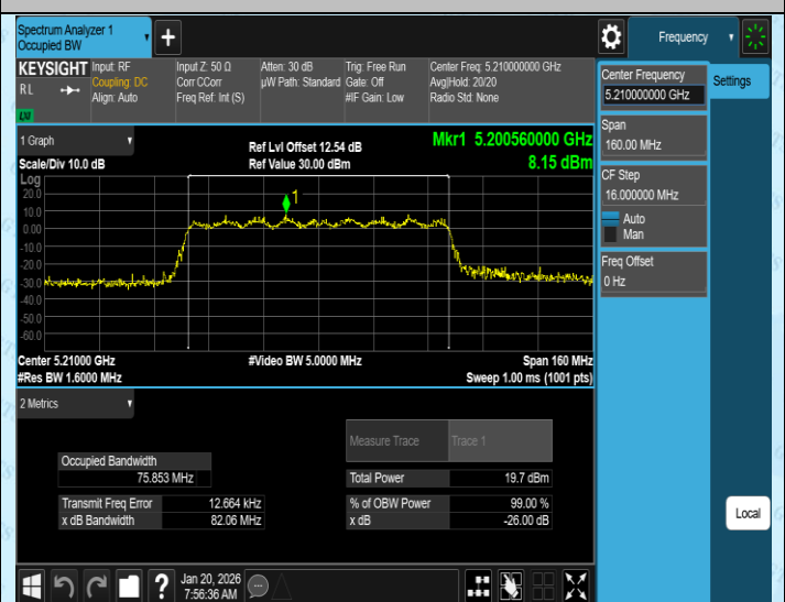
11AC80SISO-Ant4-5210
