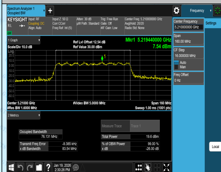
11AC80SISO-Ant3-5210
