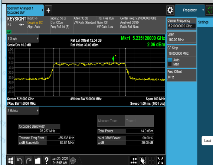
11AC80MIMO-Ant3-5210
