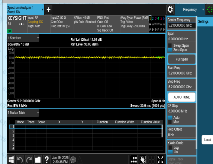
NTNV-11AC80SISO-Ant3-5210
