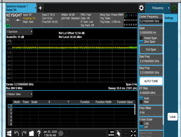
NTNV-11AC80SISO-Ant4-5210
