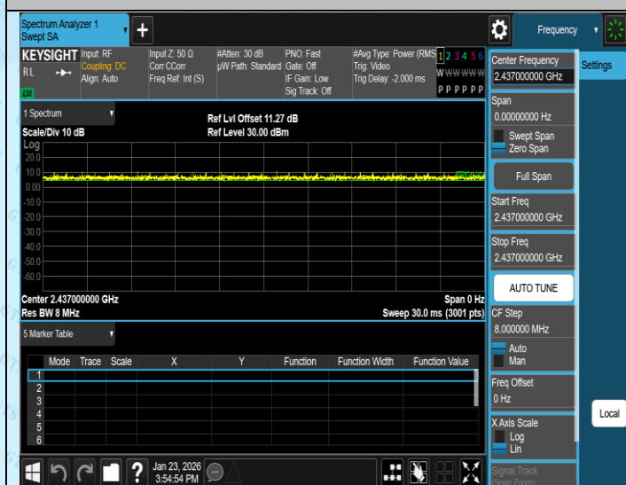
NTNV-11N20MIMO-Ant1-2437
