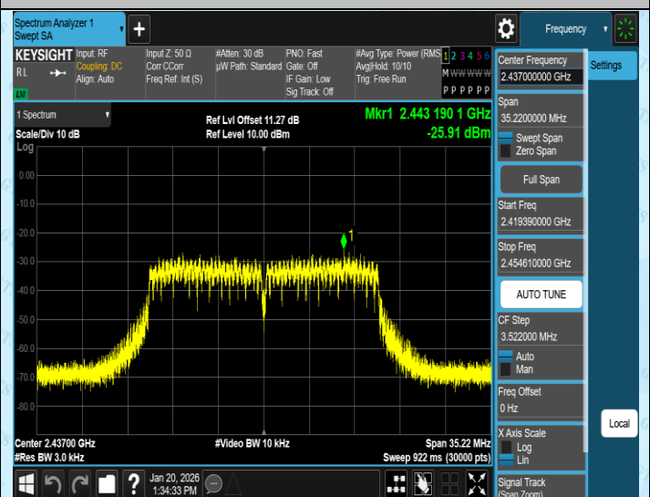
11N20MIMO-Ant4-2437-PASS
