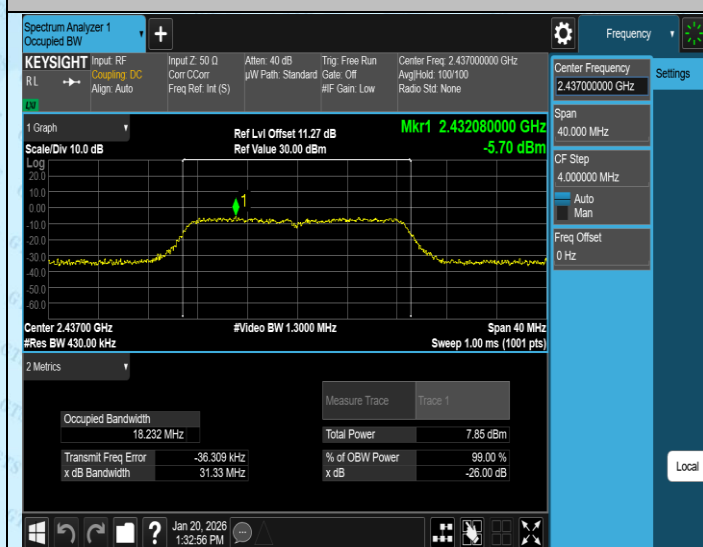
11N20MIMO-Ant3-2437
