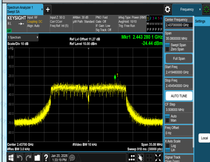
11N20MIMO-Ant3-2437-PASS
