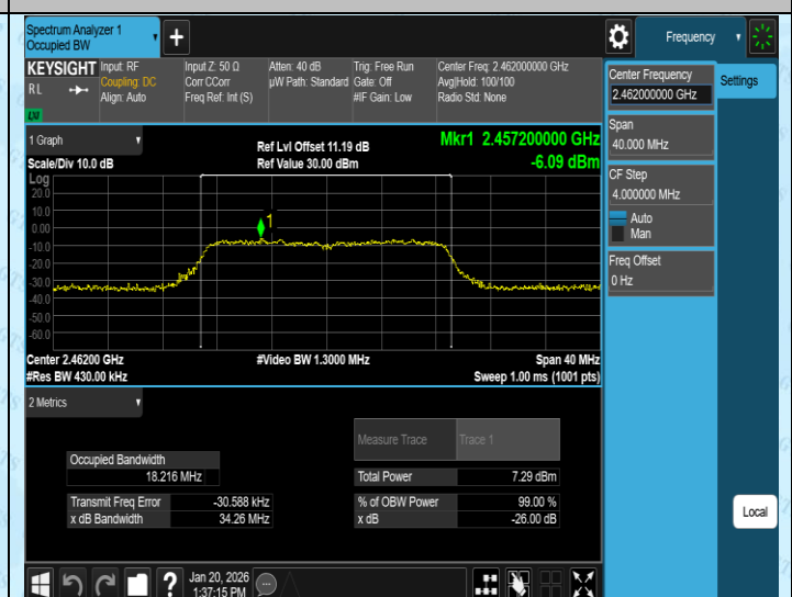
11N20MIMO-Ant4-2462
