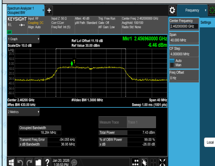
11N20MIMO-Ant3-2462
