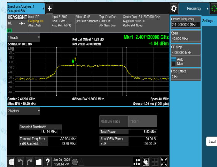
11N20MIMO-Ant3-2412
