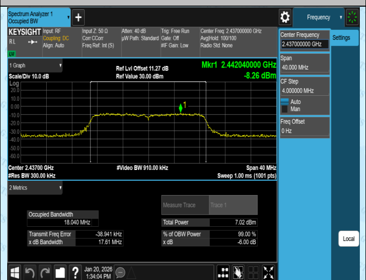
11N20MIMO-Ant4-2437-PASS
