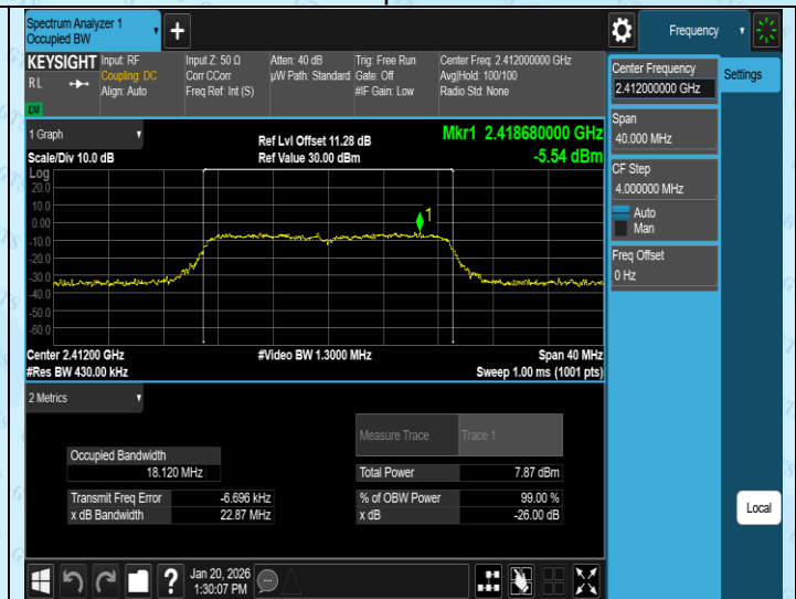
11N20MIMO-Ant4-2412
