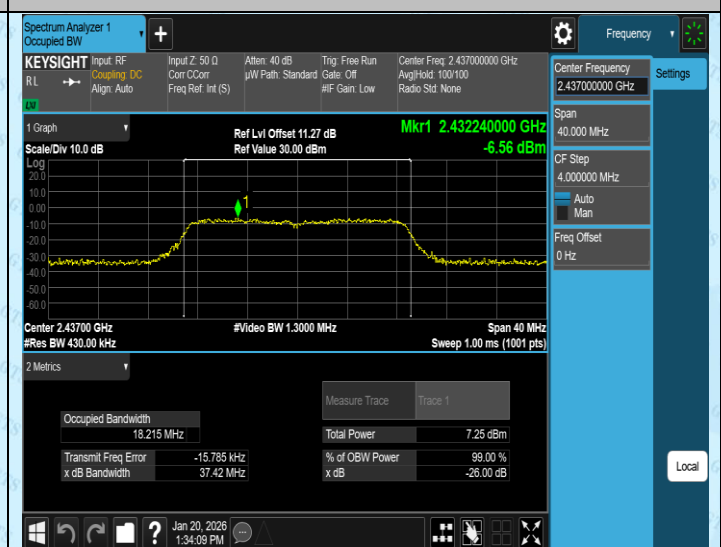
11N20MIMO-Ant4-2437
