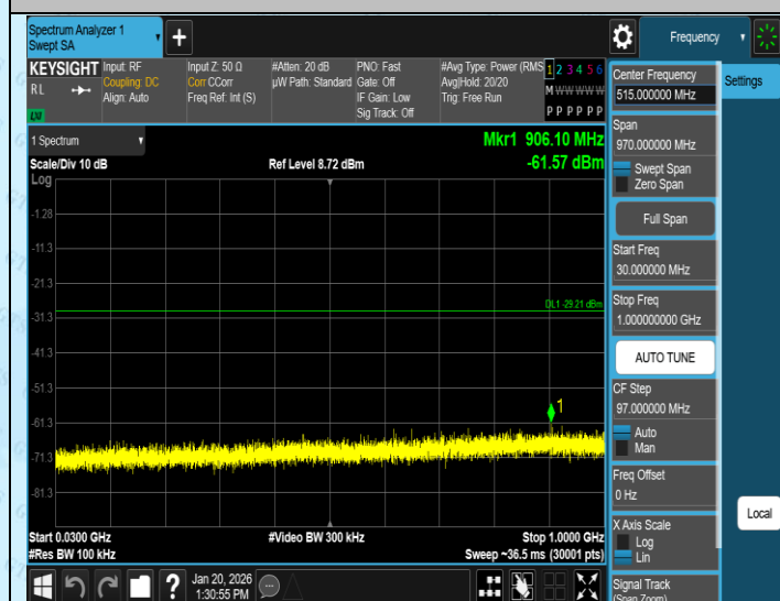
11N20MIMO-Ant4-2412-30~1000-PASS
