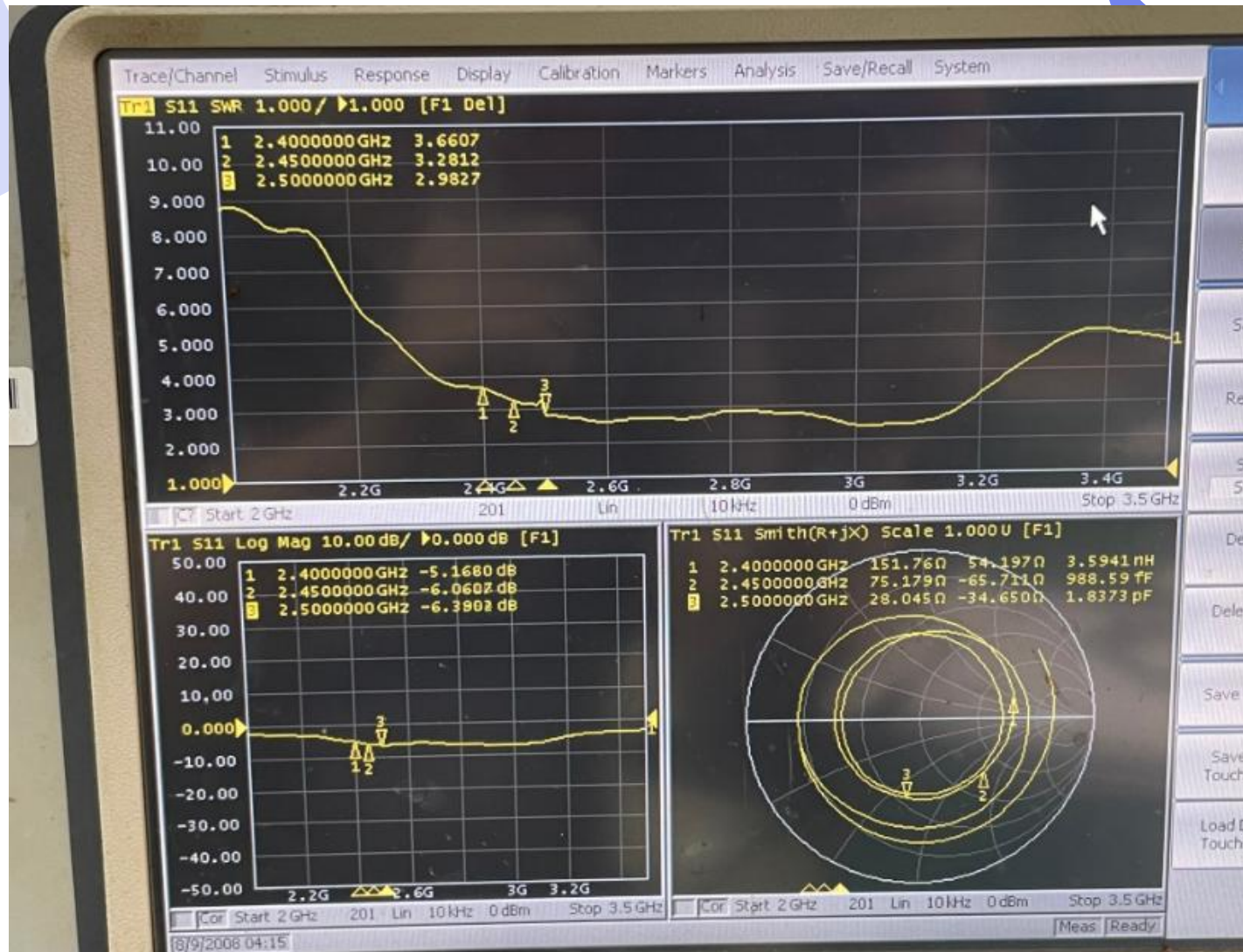
天线S11
