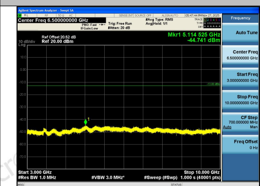
Band26(824-849)-1.4MHz-QPSK-26797-1RB#0-3 000~10000-PASS
