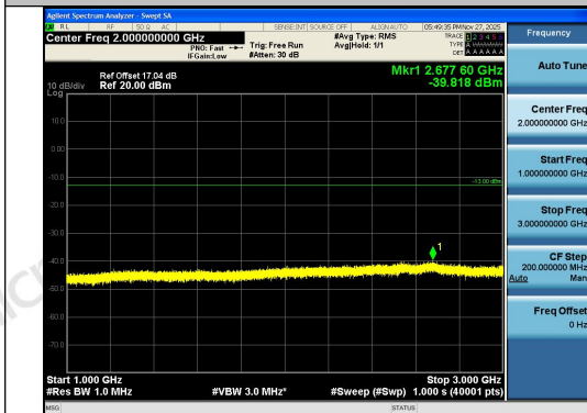
Band26(824-849)-1.4MHz-QPSK-26797-1RB#5-1 000~3000-PASS
