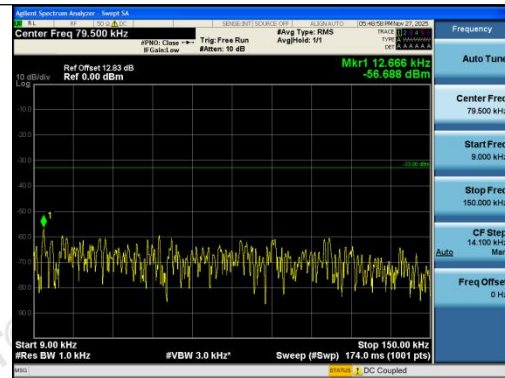
Band26(824-849)-1.4MHz-QPSK-26797-1RB#5-0. 009~0.15-PASS
