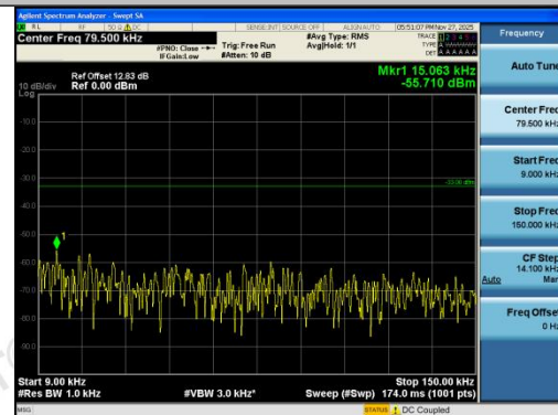
Band26(824-849)-1.4MHz-QPSK-26797-6RB#0-0. 009~0.15-PASS
