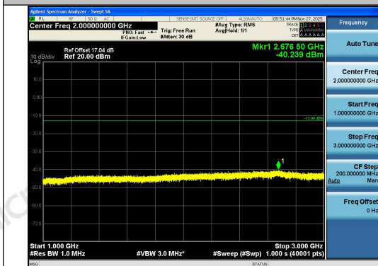
Band26(824-849)-1.4MHz-QPSK-26797-6RB#0-1 000~3000-PASS
