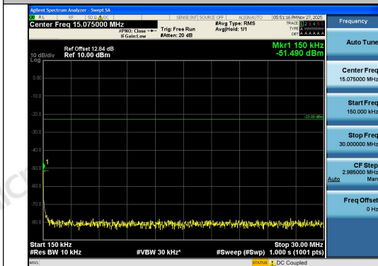
Band26(824-849)-1.4MHz-QPSK-26797-6RB#0-0. 15~30-PASS
