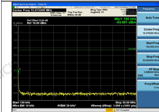
Band26(824-849)-1.4MHz-QPSK-26915-6RB#0-0. 15~30-PASS
