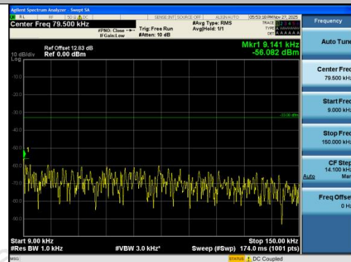
Band26(824-849)-1.4MHz-QPSK-26915-1RB#0-0. 009~0.15-PASS
