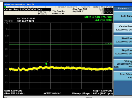
Band26(824-849)-1.4MHz-QPSK-26797-6RB#0-3 000~10000-PASS
