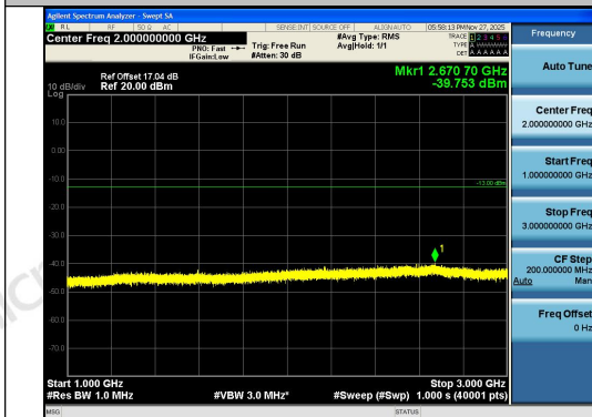
Band26(824-849)-1.4MHz-QPSK-26915-6RB#0-1 000~3000-PASS
