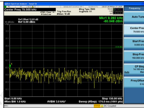
Band26(824-849)-1.4MHz-QPSK-26915-6RB#0-0. 009~0.15-PASS
