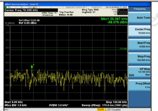
Band26(824-849)-3MHz-QPSK-26805-15RB#0-0. 009~0.15-PASS
