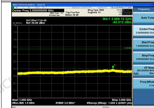
Band26(824-849)-3MHz-QPSK-26805-1RB#14-10 00~3000-PASS
