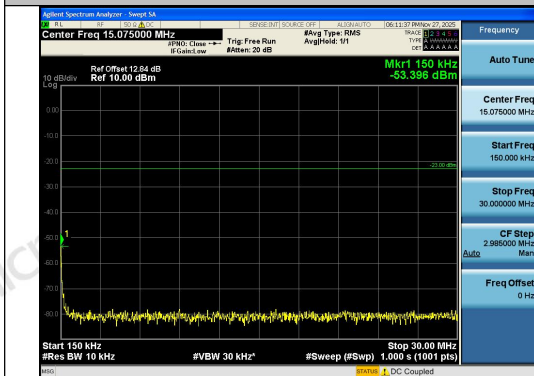
Band26(824-849)-3MHz-QPSK-26805-1RB#14-0. 15~30-PASS
