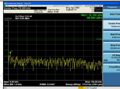
Band26(824-849)-3MHz-QPSK-26805-1RB#14-0. 009~0.15-PASS
