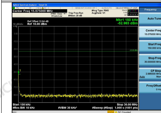
Band26(824-849)-3MHz-QPSK-26805-15RB#0-0. 15~30-PASS
