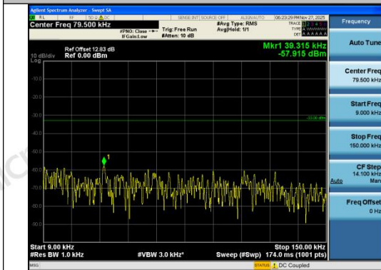
Band26(824-849)-3MHz-16QAM-27025-1RB#0-0. 009~0.15-PASS
