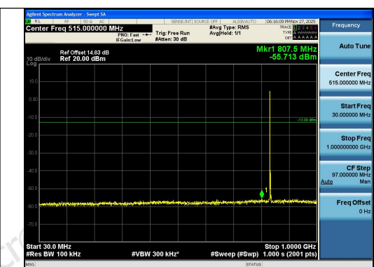
Band26(824-849)-3MHz-QPSK-26915-1RB#0-30~ 1000-PASS
