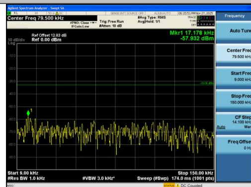
Band26(824-849)-3MHz-QPSK-26915-1RB#0-0.0 09~0.15-PASS
