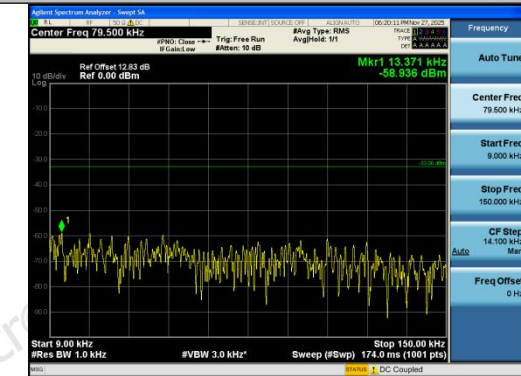
Band26(824-849)-3MHz-QPSK-26915-15RB#0-0. 009~0.15-PASS
