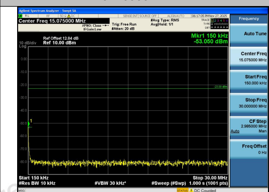
Band26(824-849)-3MHz-16QAM-26915-1RB#0-0. 15~30-PASS
