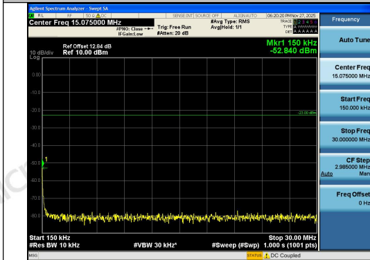
Band26(824-849)-3MHz-QPSK-26915-15RB#0-0. 15~30-PASS
