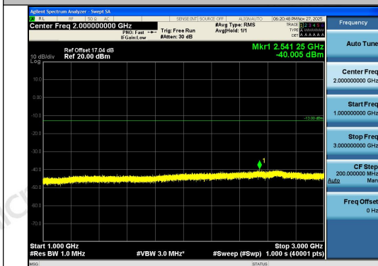
Band26(824-849)-3MHz-QPSK-26915-15RB#0-10 00~3000-PASS
