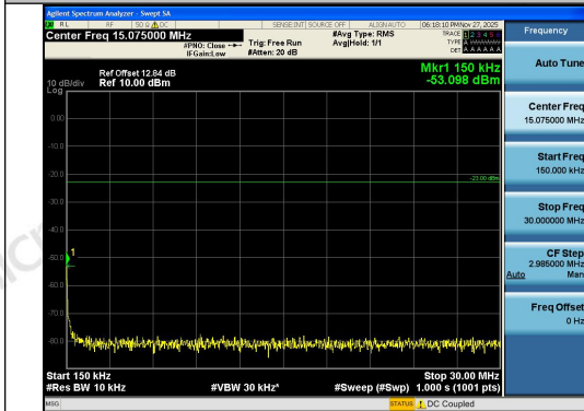
Band26(824-849)-3MHz-QPSK-26915-1RB#14-0. 15~30-PASS
