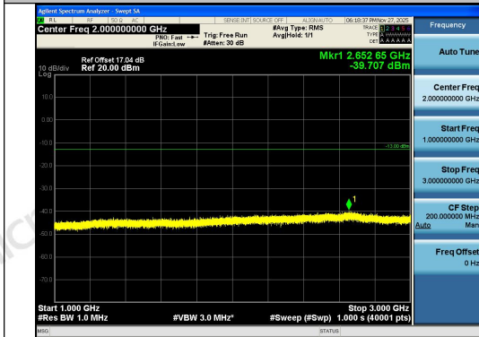
Band26(824-849)-3MHz-QPSK-26915-1RB#14-10 00~3000-PASS
