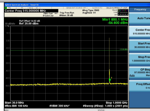
Band26(824-849)-3MHz-QPSK-27025-1RB#0-30~ 1000-PASS
