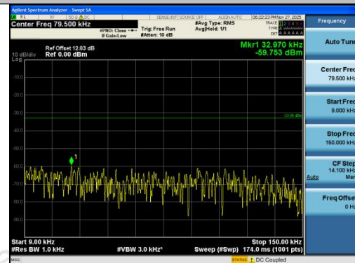
Band26(824-849)-3MHz-QPSK-27025-1RB#0-0.0 09~0.15-PASS
