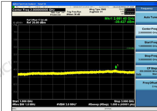
Band26(824-849)-3MHz-QPSK-27025-1RB#0-100 0~3000-PASS
