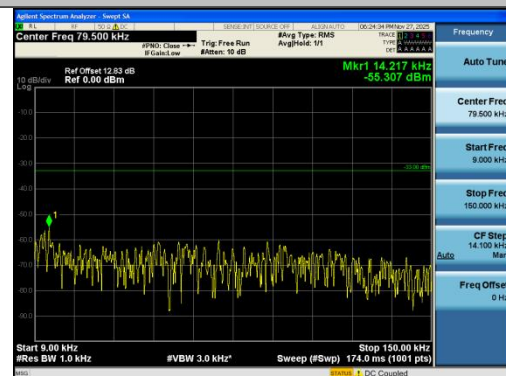
Band26(824-849)-3MHz-QPSK-27025-1RB#14-0. 009~0.15-PASS
