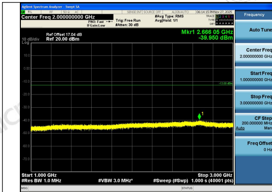
Band26(824-849)-3MHz-QPSK-26805-15RB#0-10 00~3000-PASS
