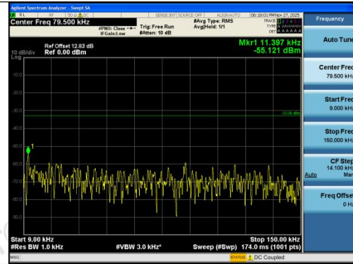
Band26(824-849)-3MHz-QPSK-26915-1RB#14-0. 009~0.15-PASS
