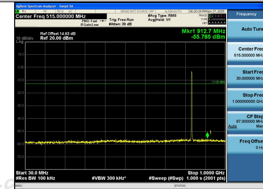
Band26(824-849)-3MHz-QPSK-26915-15RB#0-30 ~1000-PASS
