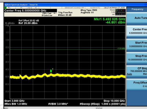
Band26(824-849)-3MHz-QPSK-27025-15RB#0-30 00~10000-PASS
