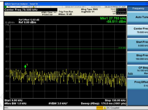
Band26(824-849)-3MHz-QPSK-27025-15RB#0-0. 009~0.15-PASS
