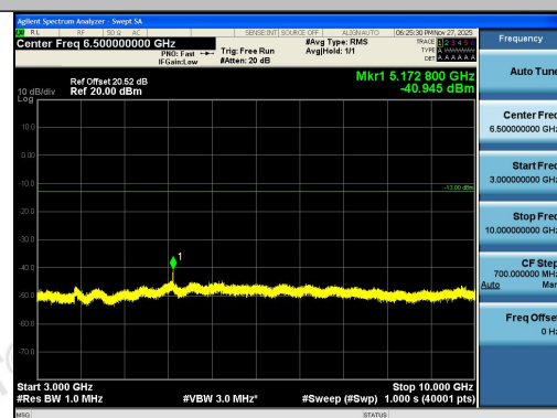
Band26(824-849)-3MHz-QPSK-27025-1RB#14-30 00~10000-PASS
