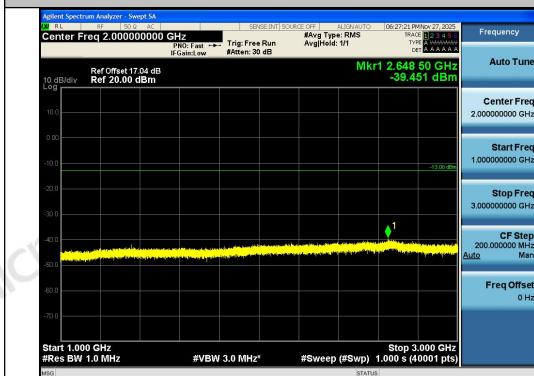
Band26(824-849)-3MHz-QPSK-27025-15RB#0-10 00~3000-PASS
