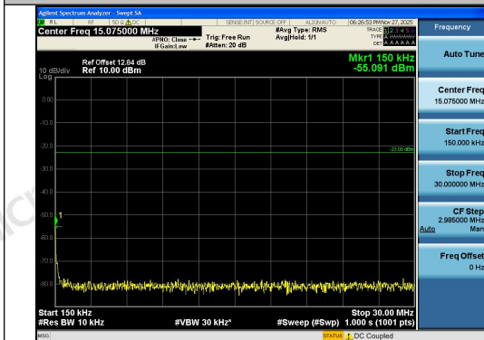
Band26(824-849)-3MHz-QPSK-27025-15RB#0-0. 15~30-PASS
