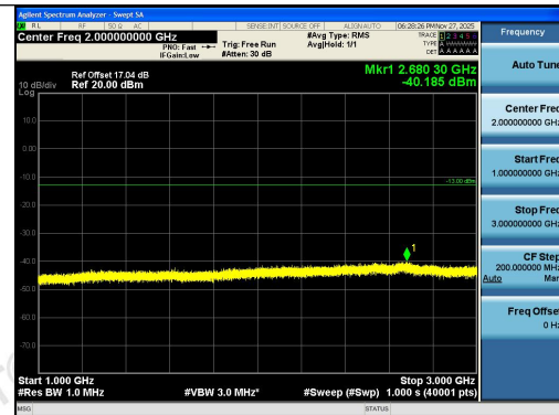
Band26(824-849)-3MHz-16QAM-27025-15RB#0-1 000~3000-PASS
